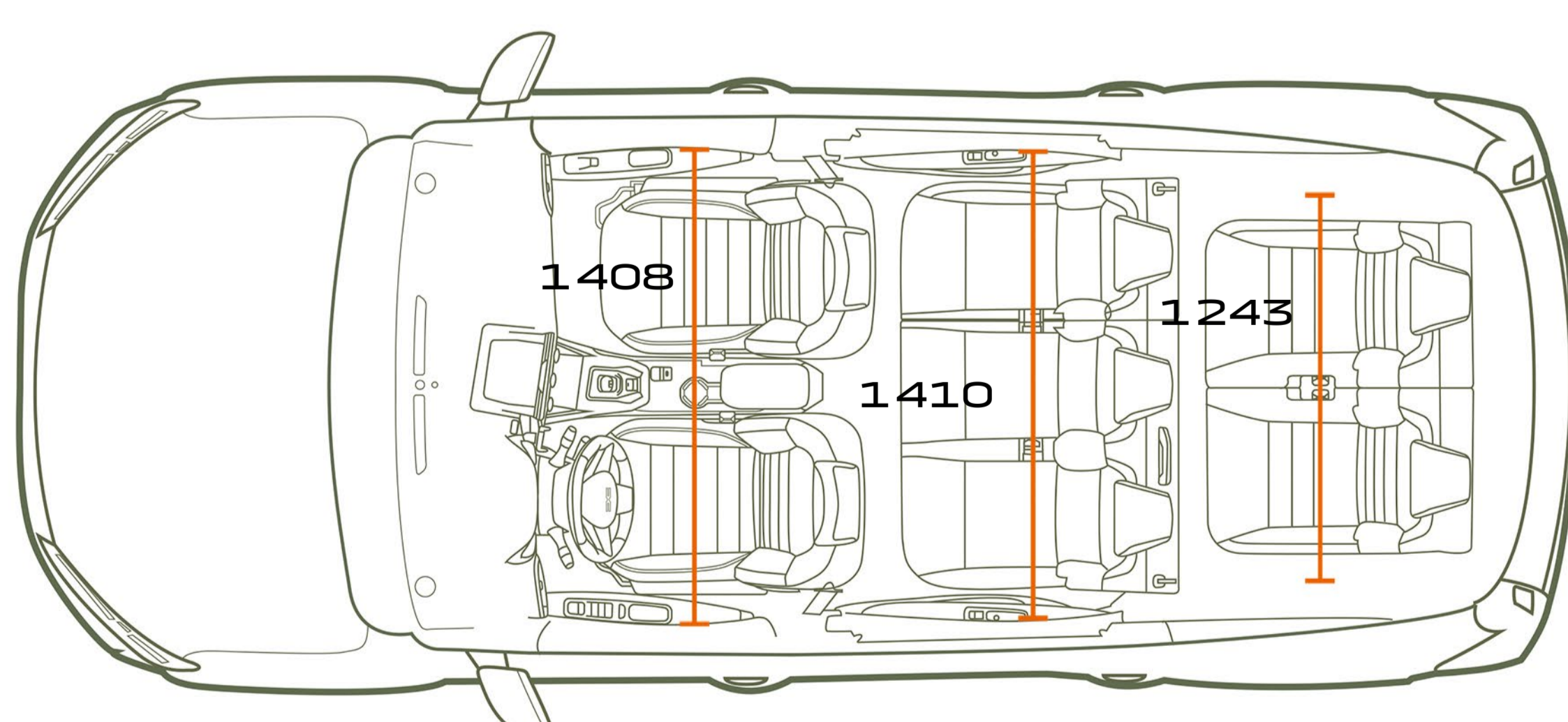
DRAUFSICHT 7-PLÄTZER
