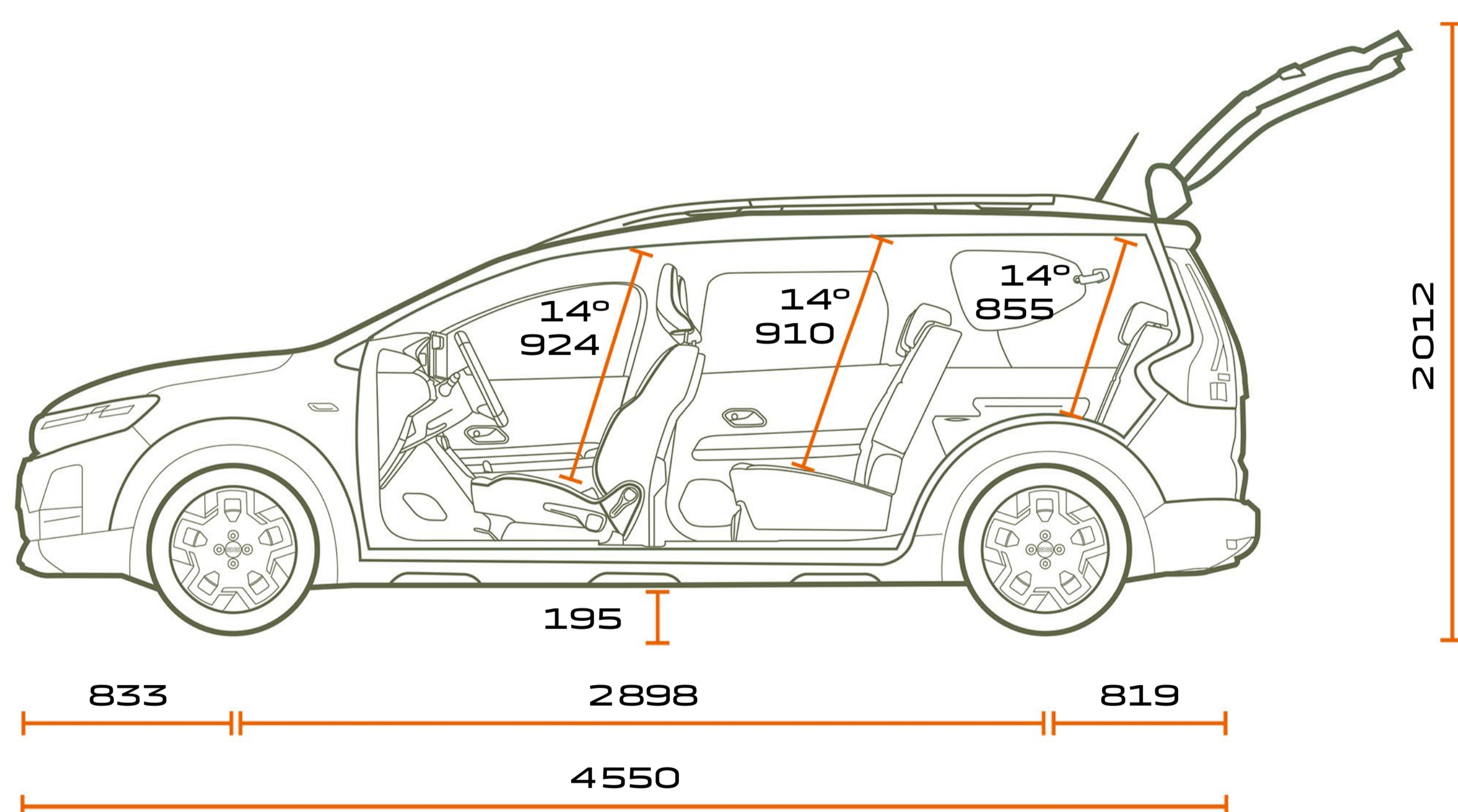
SEITENANSICHT 7-PLÄTZER
