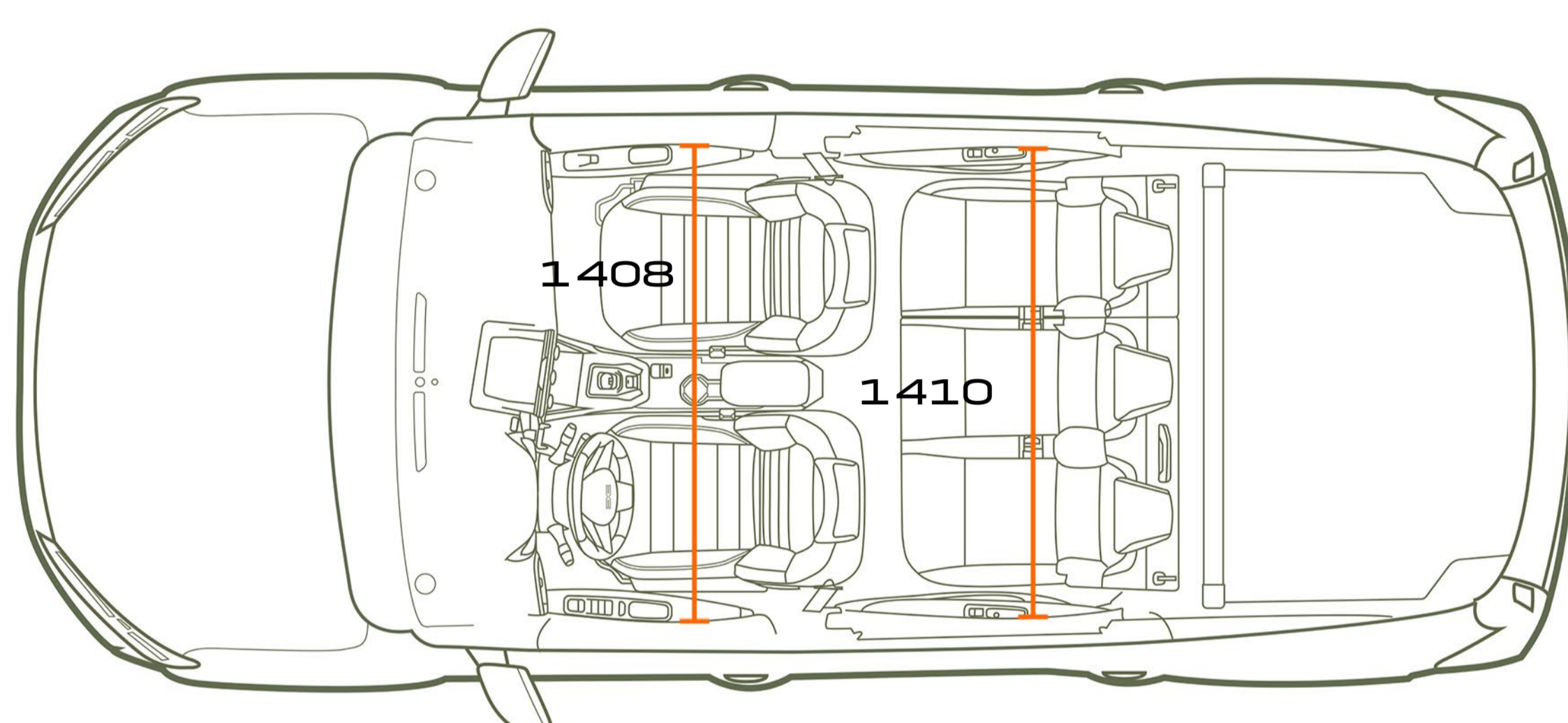
DRAUFSICHT 5-PLÄTZER
