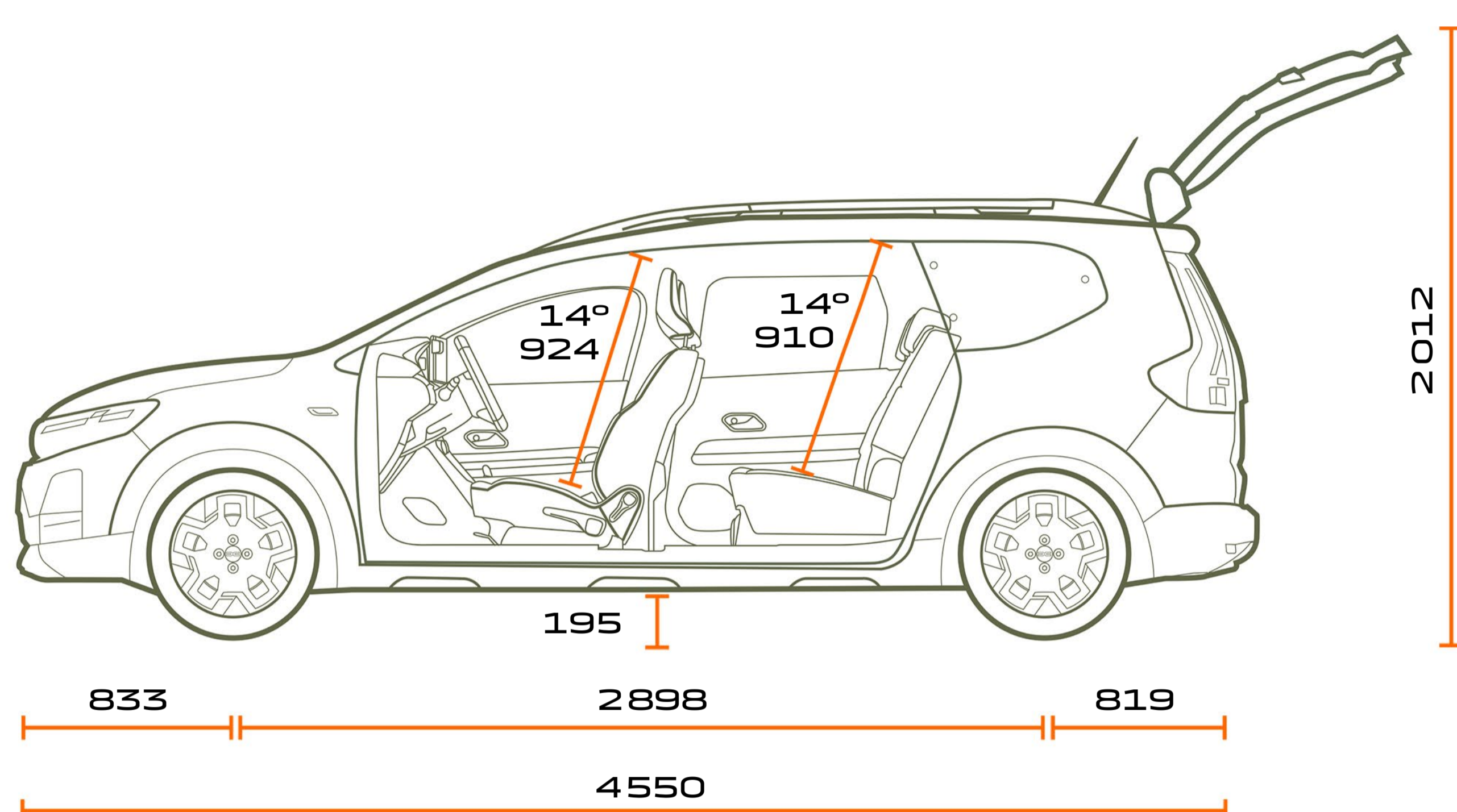
SEITENANSICHT 5-PLÄTZER
