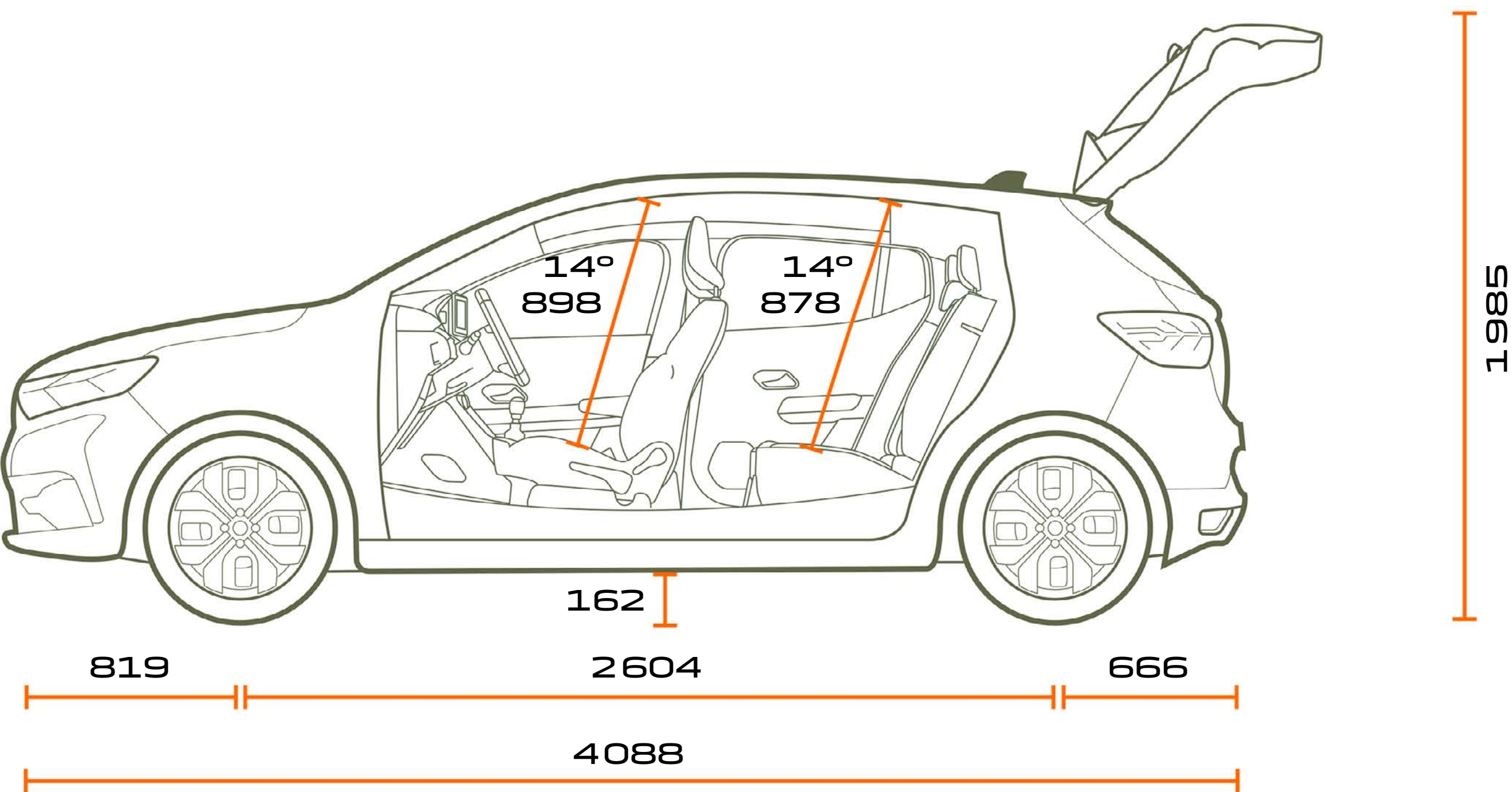
SEITENANSICHT
