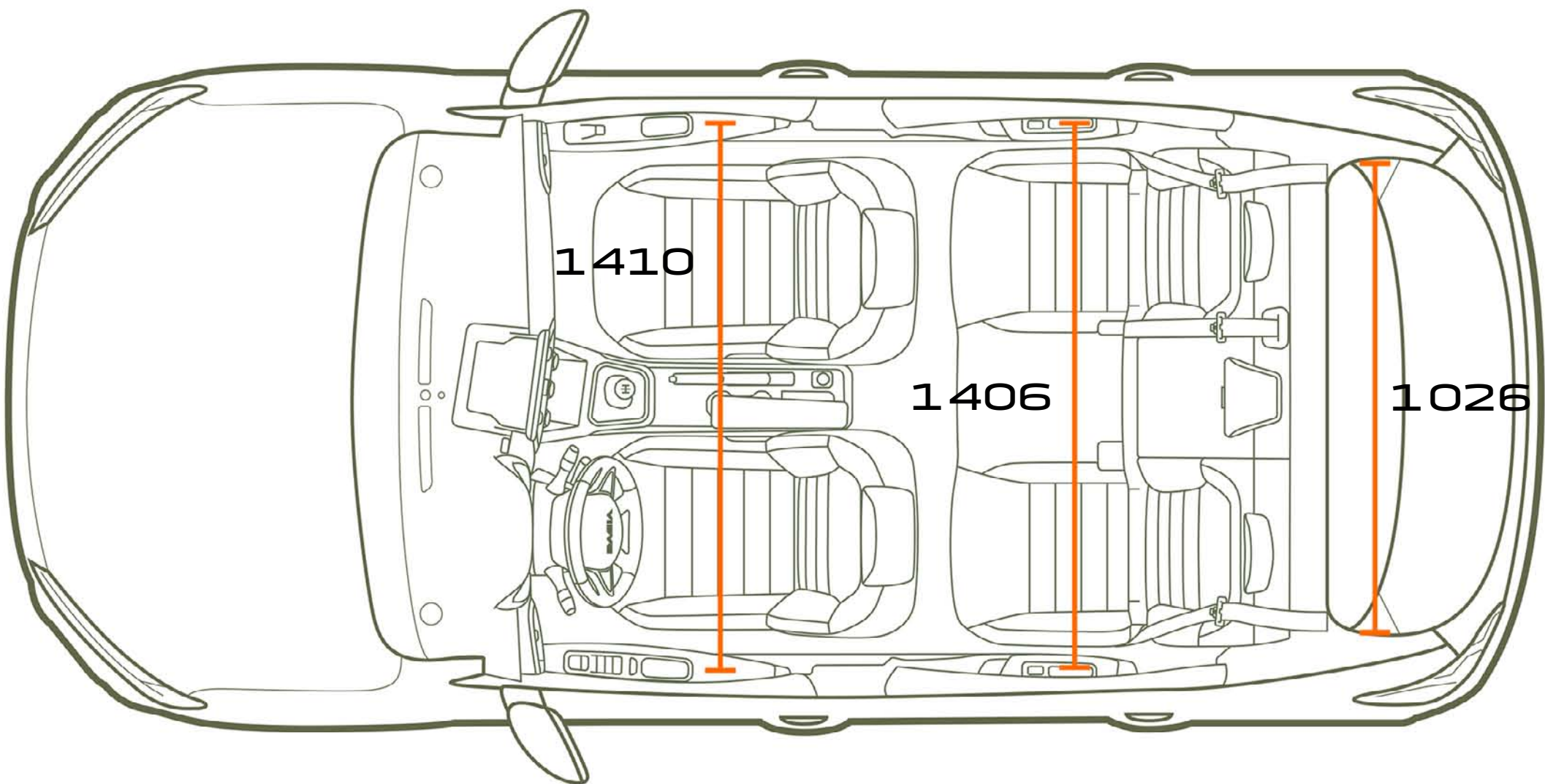
DRAUFSICHT
