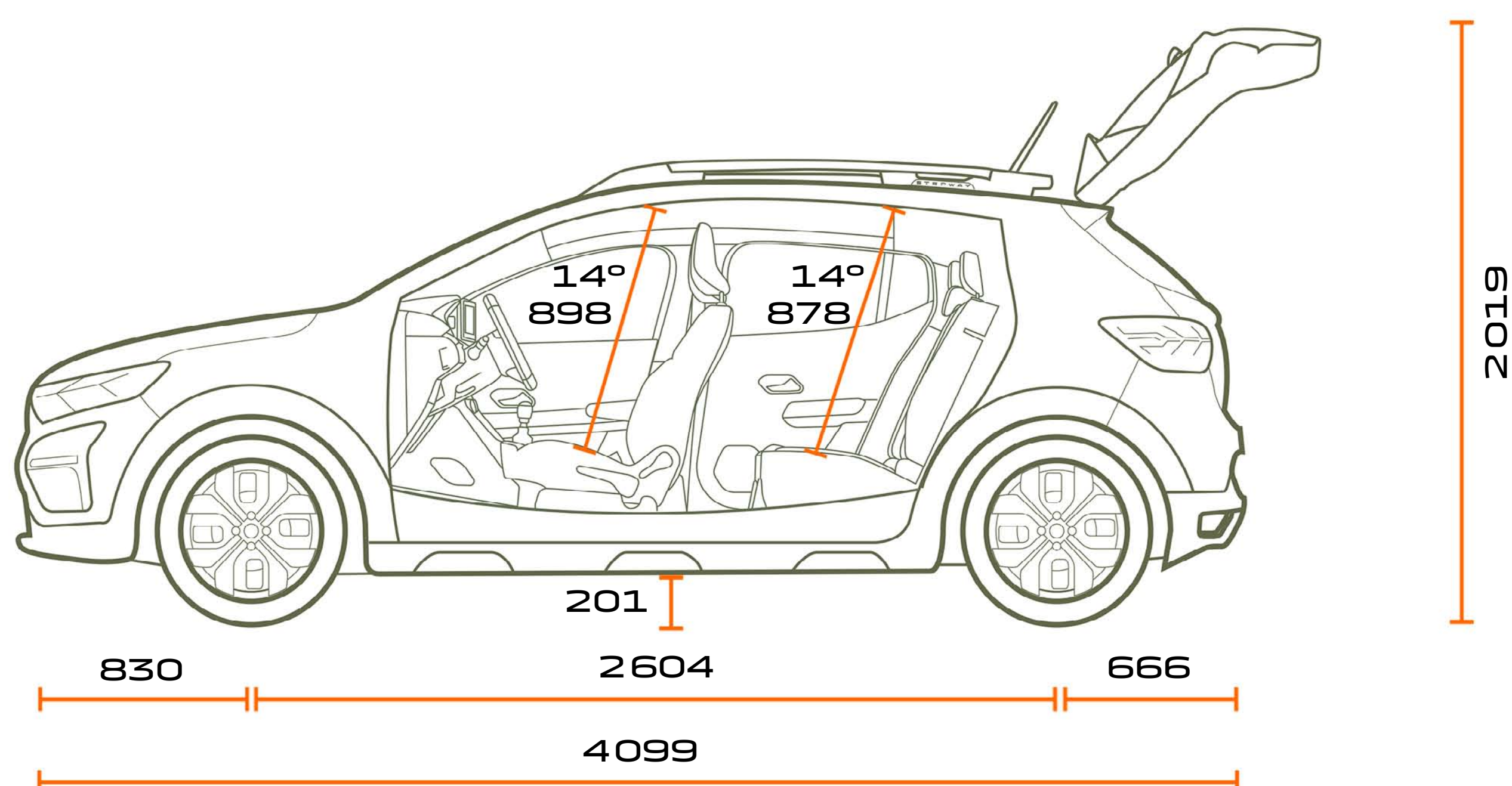
VISTA PROFILO
