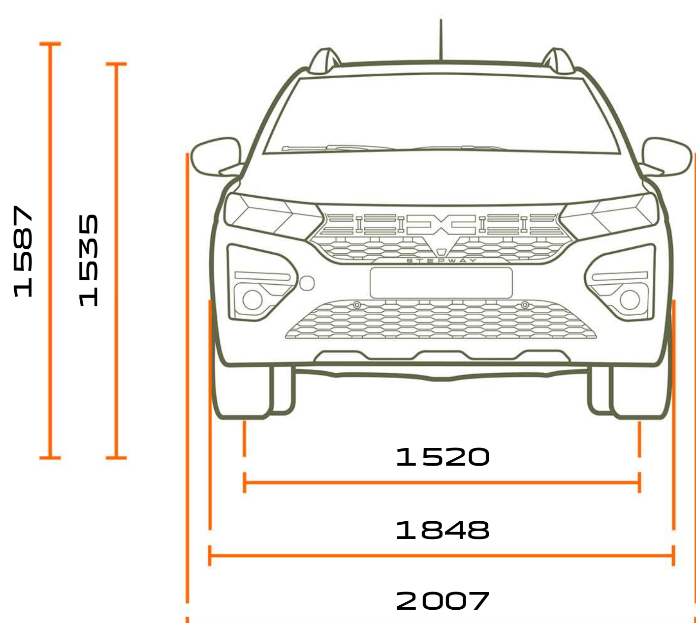
VISTA ANTERIORE
