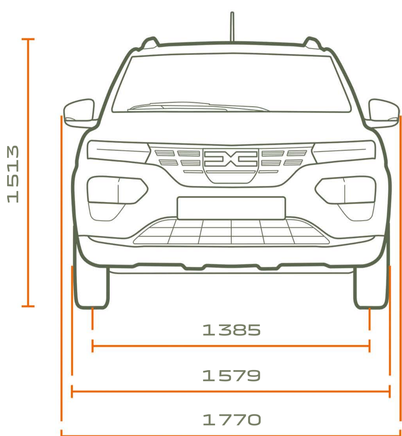
FRONTANSICHT
