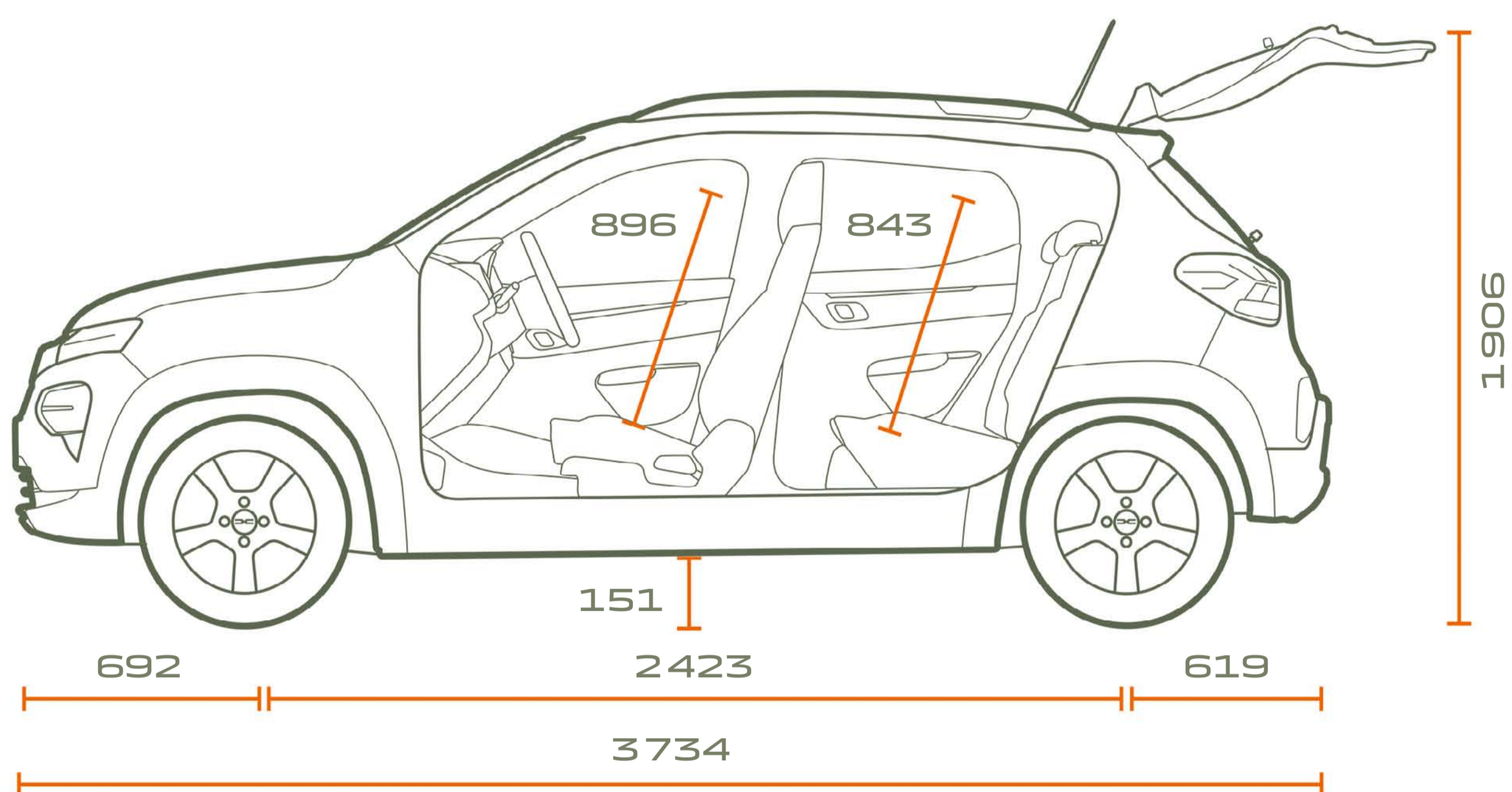
SEITENANSICHT
