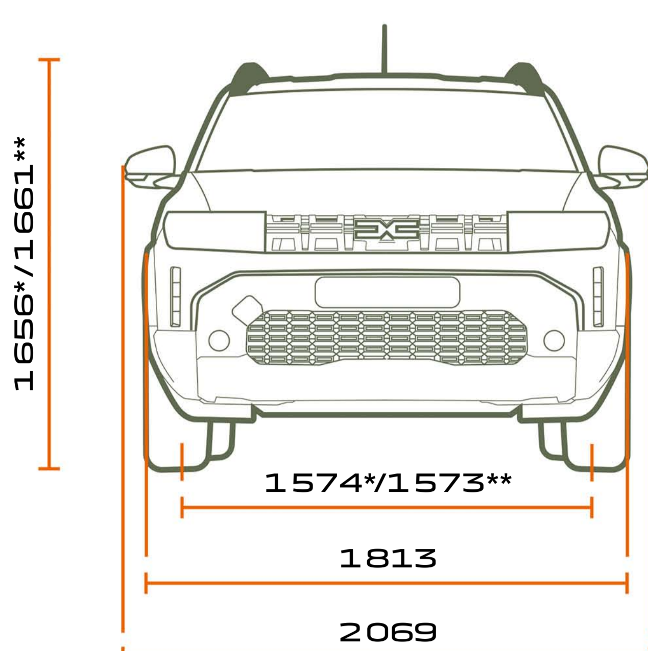
FRONTANSICHT
