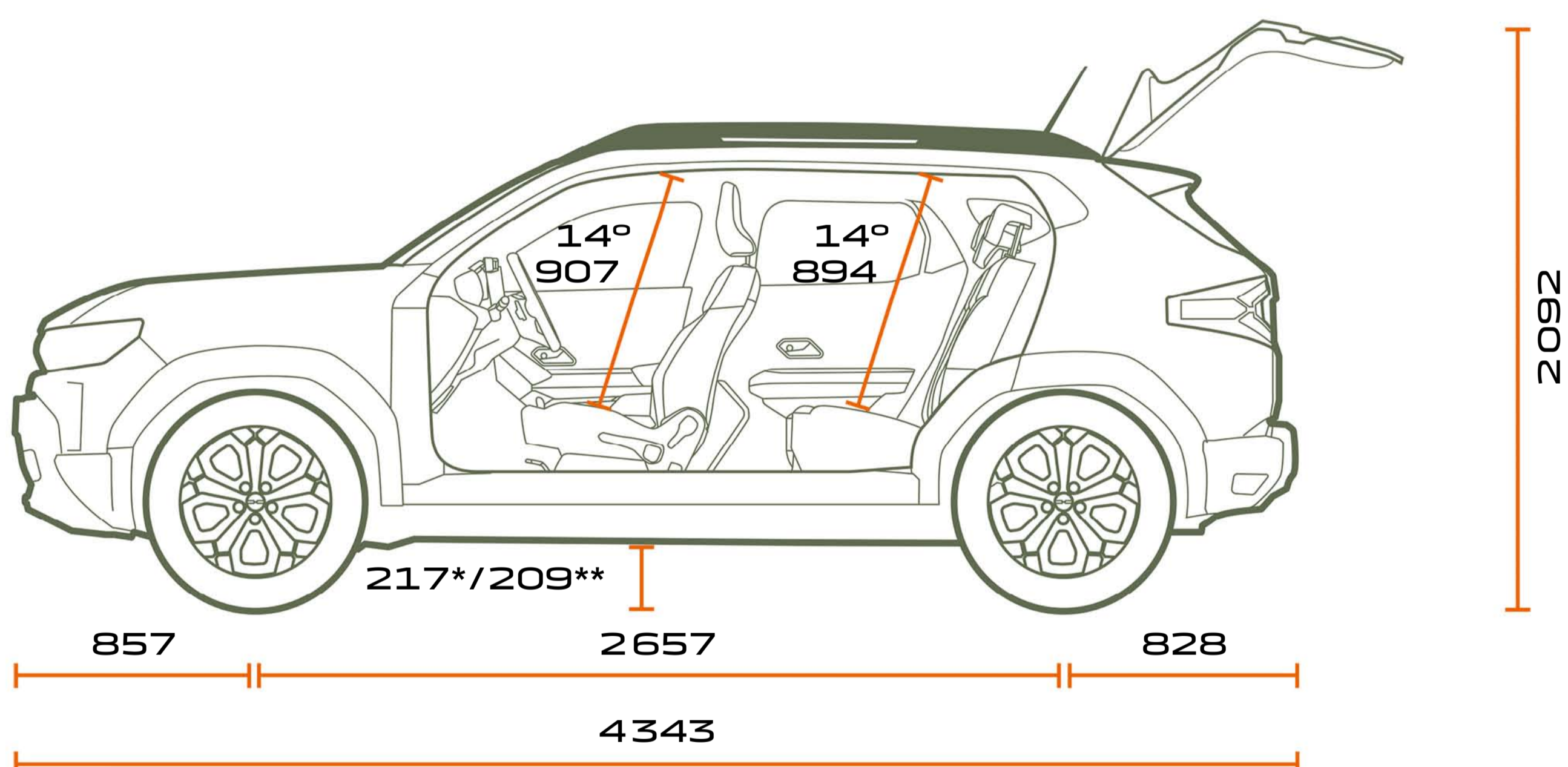
SEITENANSICHT
