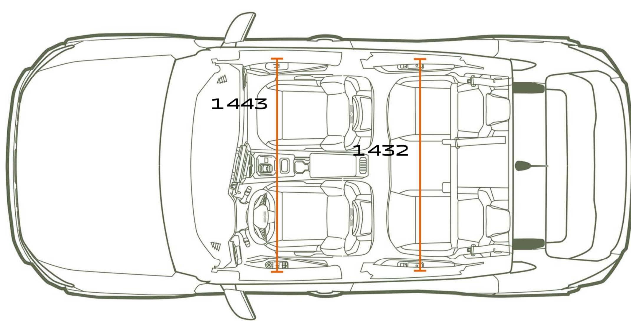
DRAUFSICHT
