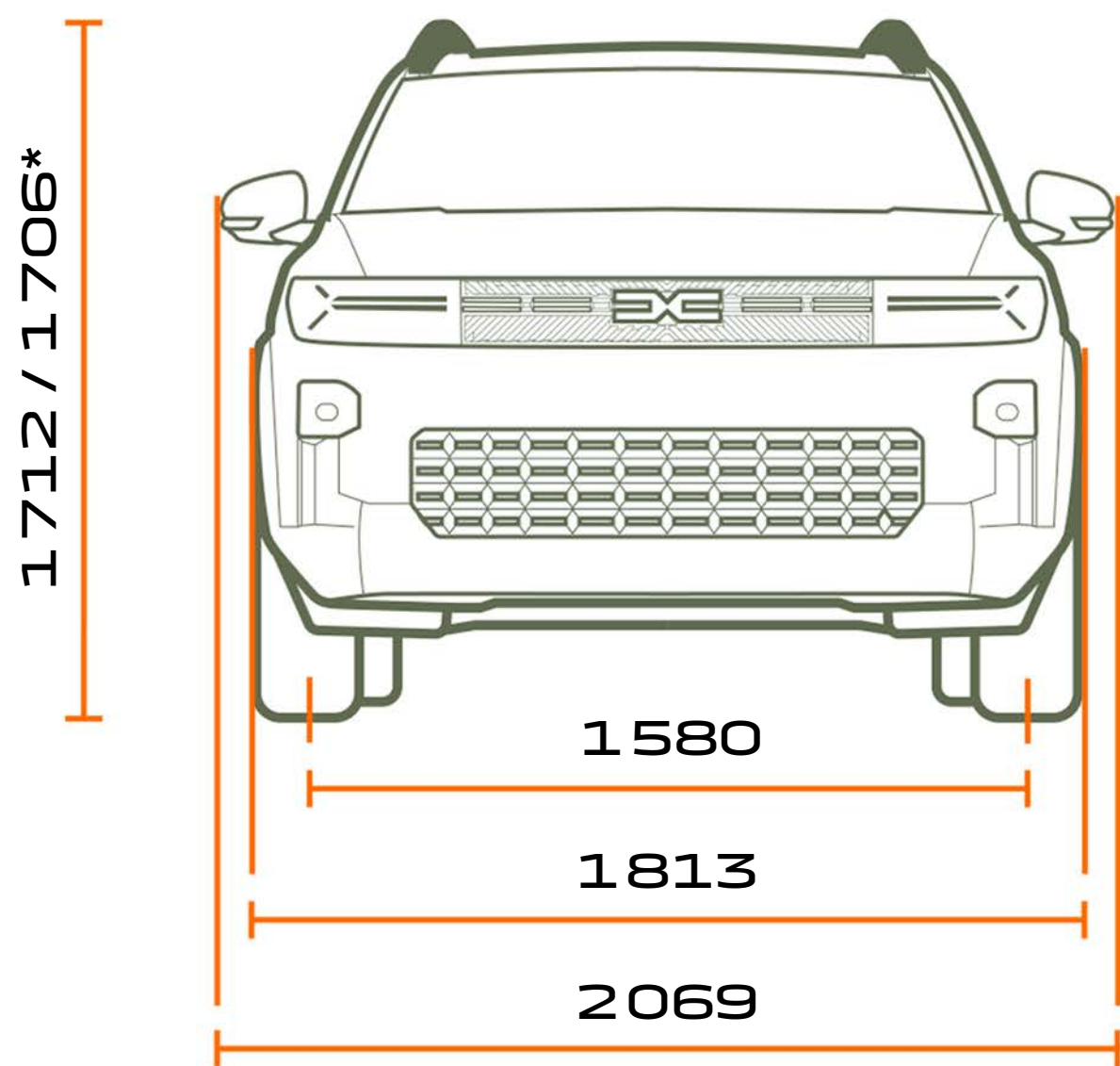
ČELNÍ POHLED
