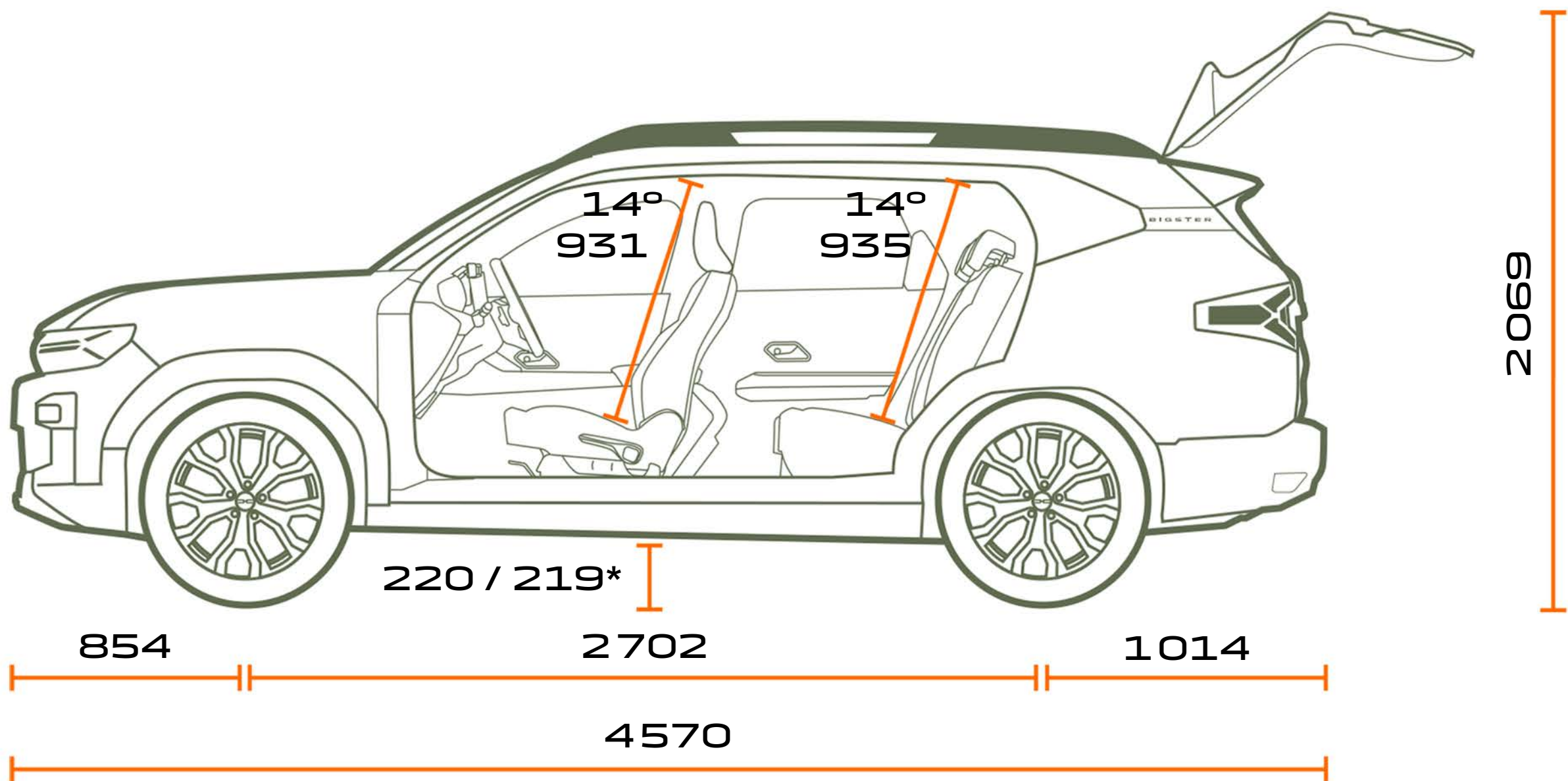
BOČNÍ POHLED
