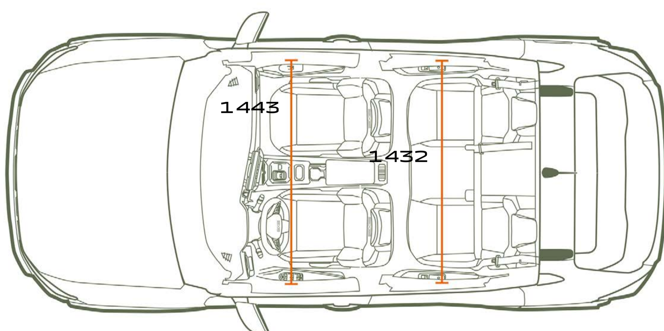
POHLED SHORA
