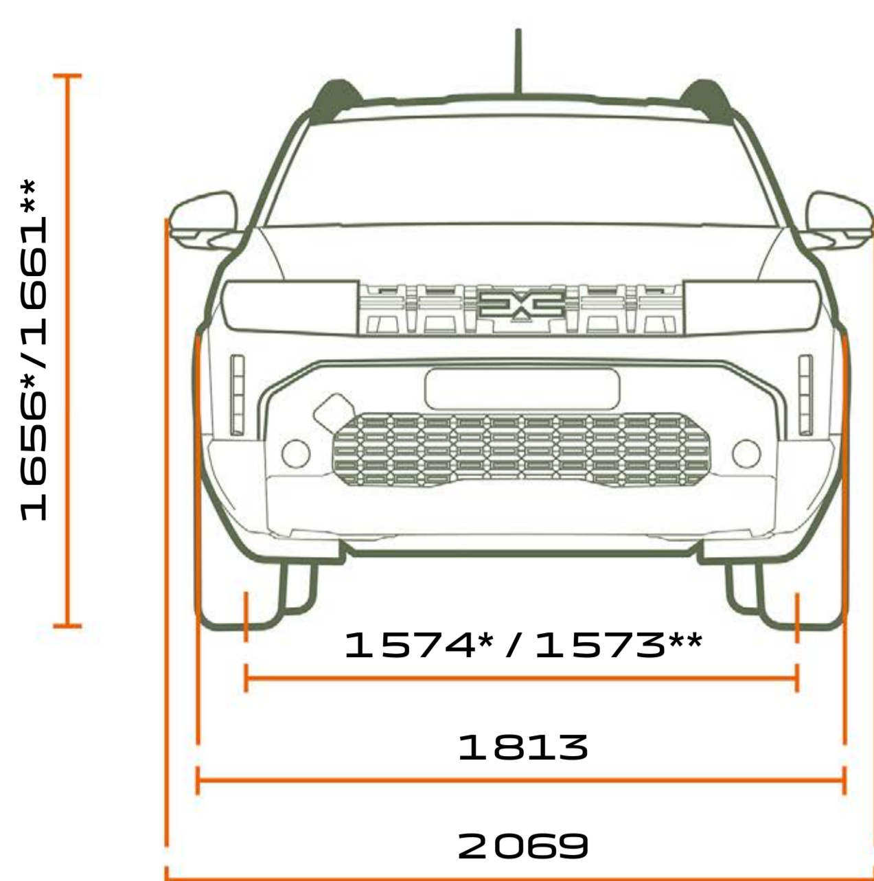
ČELNÍ POHLED
