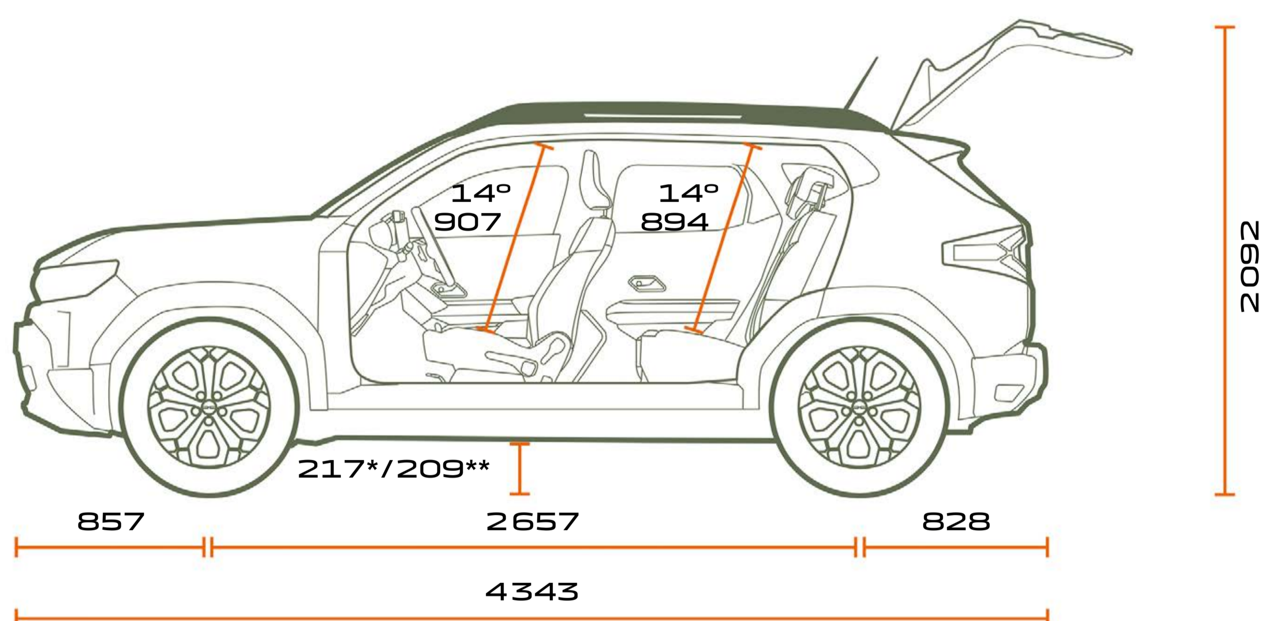
BOČNÍ POHLED
