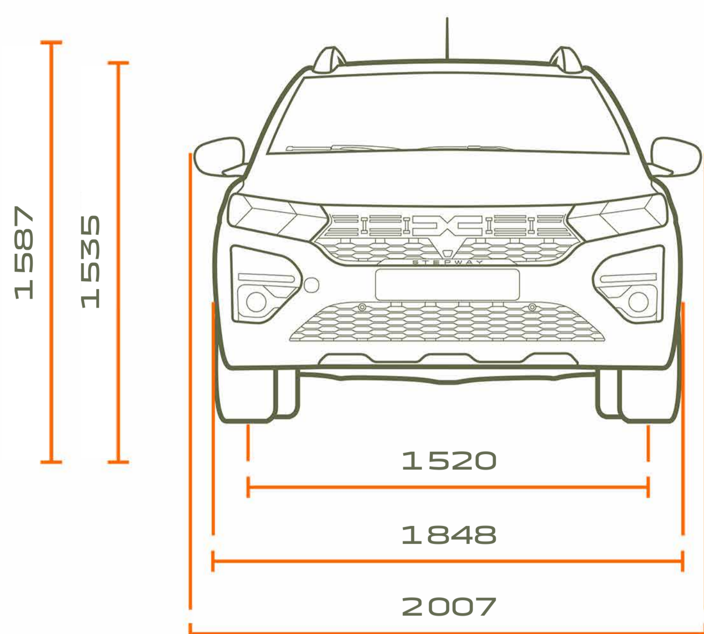
ČELNÍ POHLED
