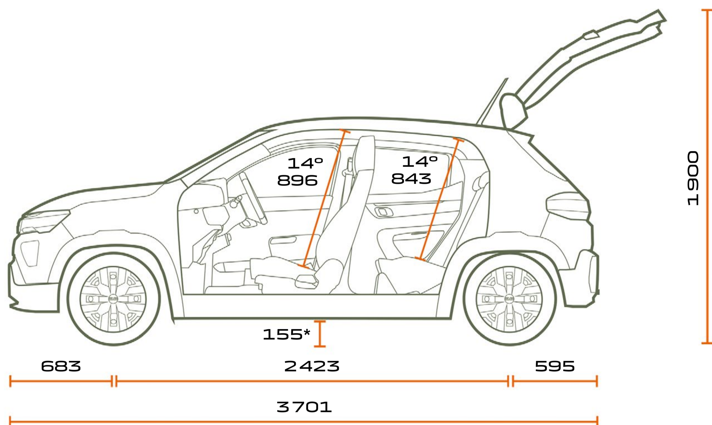
BOČNÍ POHLED
