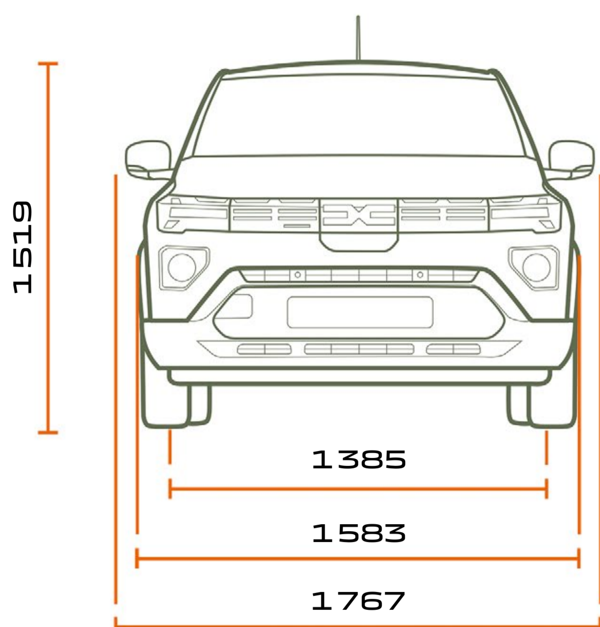
ČELNÍ POHLED
