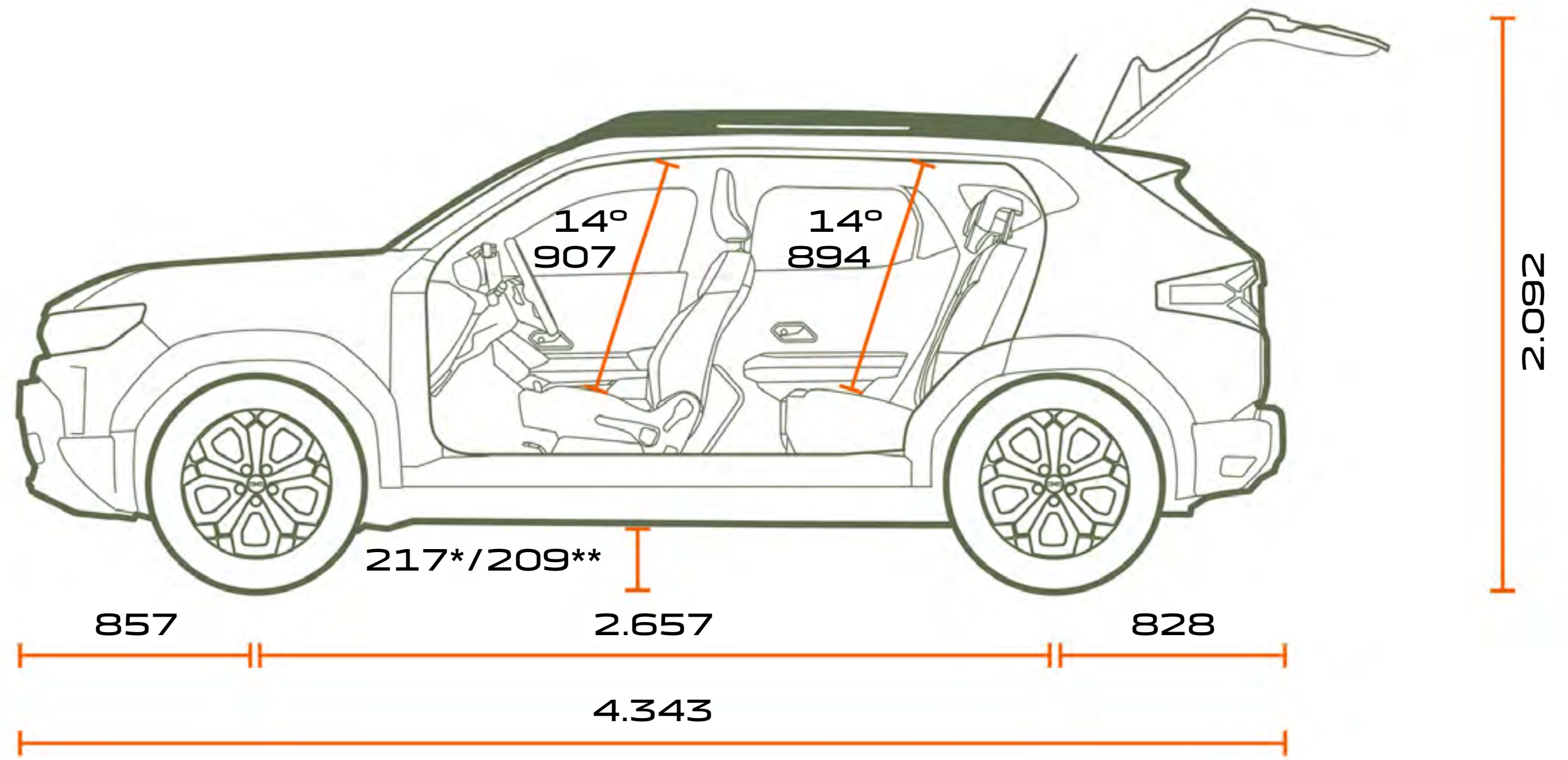
PROFILANSICHT
