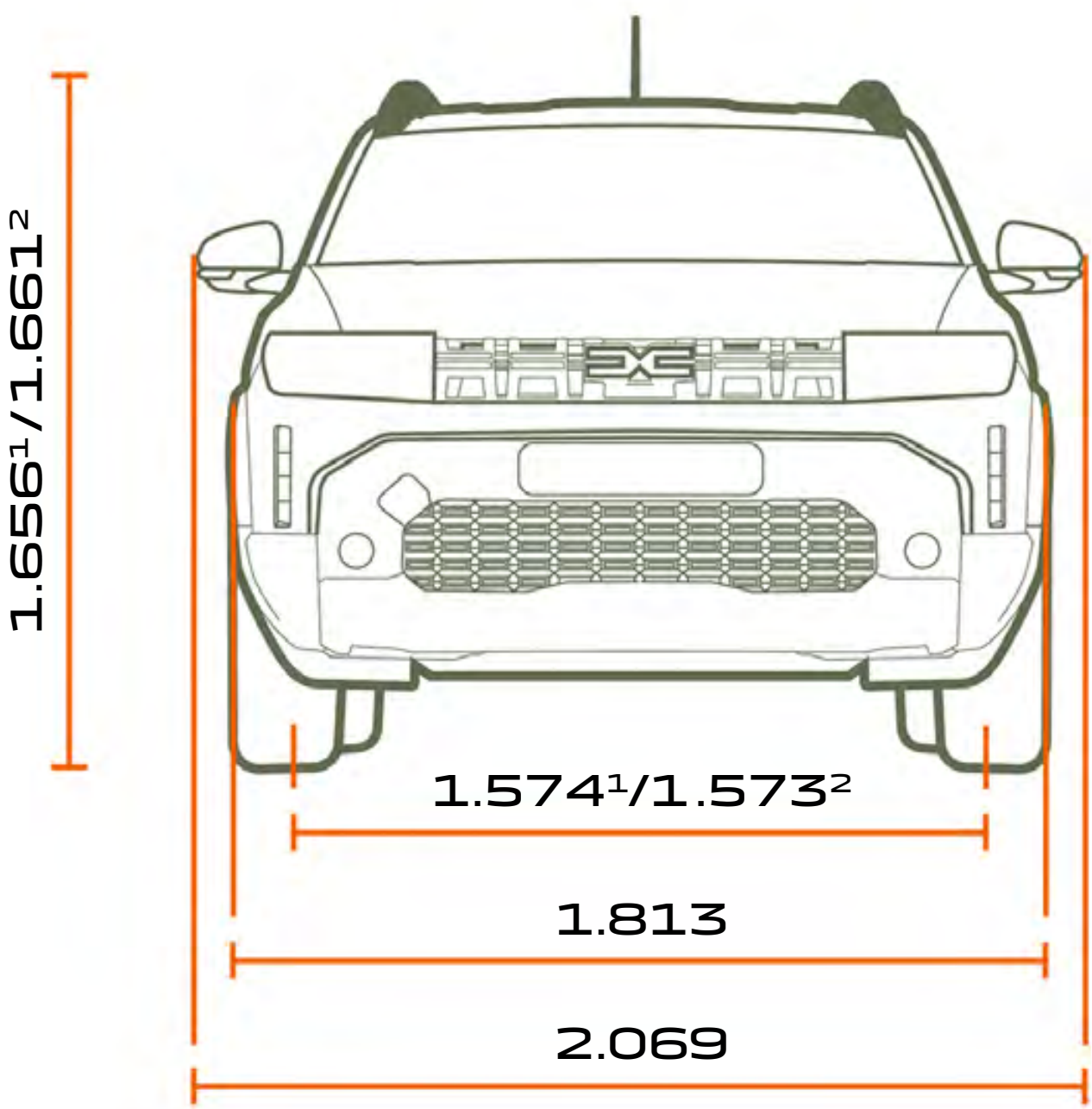
VORDERANSICHT
