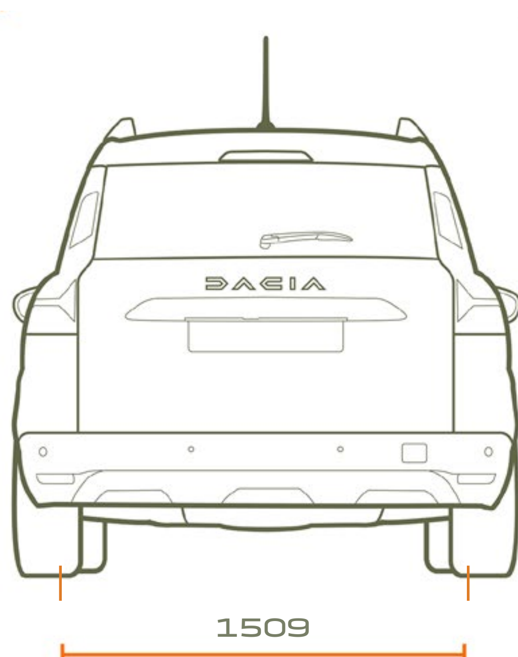
WIDOK Z TYŁU WERSJI 5- I 7-MIEJSCOWEJ
