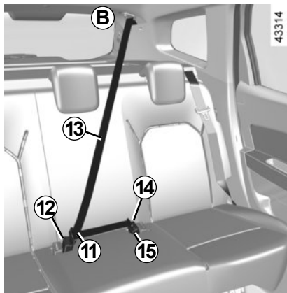
Tylny, środkowy pas bezpieczeństwa B (zależnie od wersji pojazdu)
