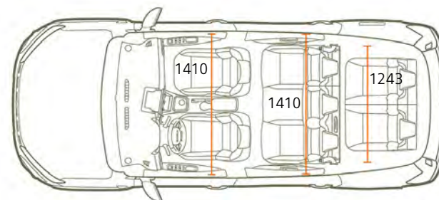
WIDOK Z GÓRY WERSJI 7-MIEJSCOWEJ
