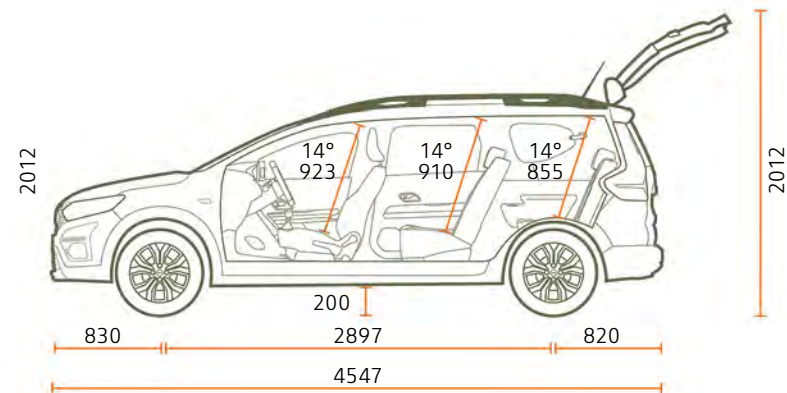
WIDOK Z BOKU WERSJI 7-MIEJSCOWEJ
