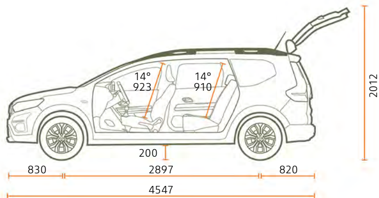
WIDOK Z BOKU WERSJI 5-MIEJSCOWEJ
