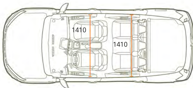
WIDOK Z GÓRY WERSJI 5-MIEJSCOWEJ
