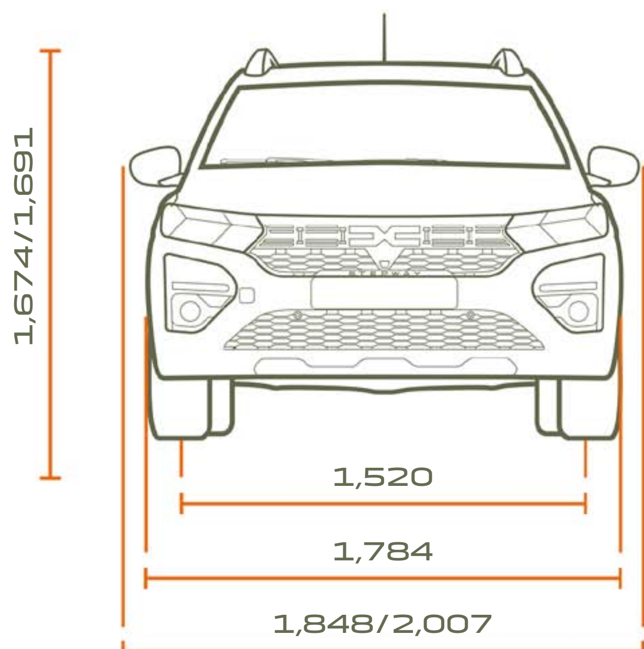
VISTA DIANTEIRA 5 E 7 LUGARES
