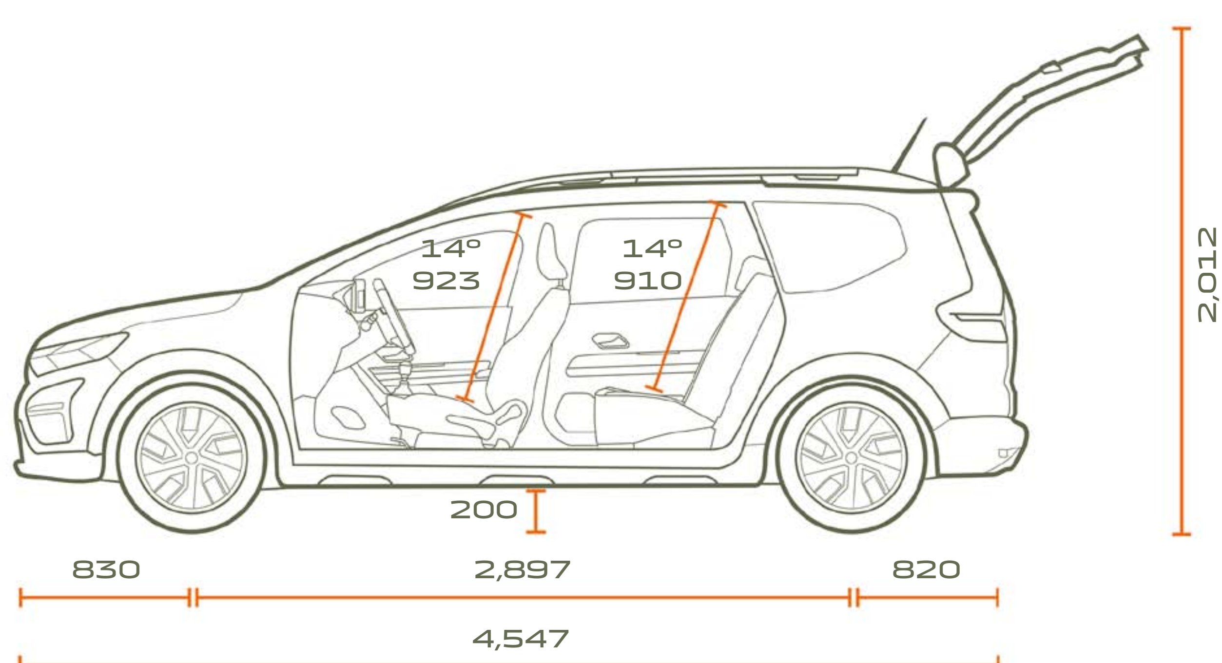
VISTA DE PERFIL 5 LUGARES
