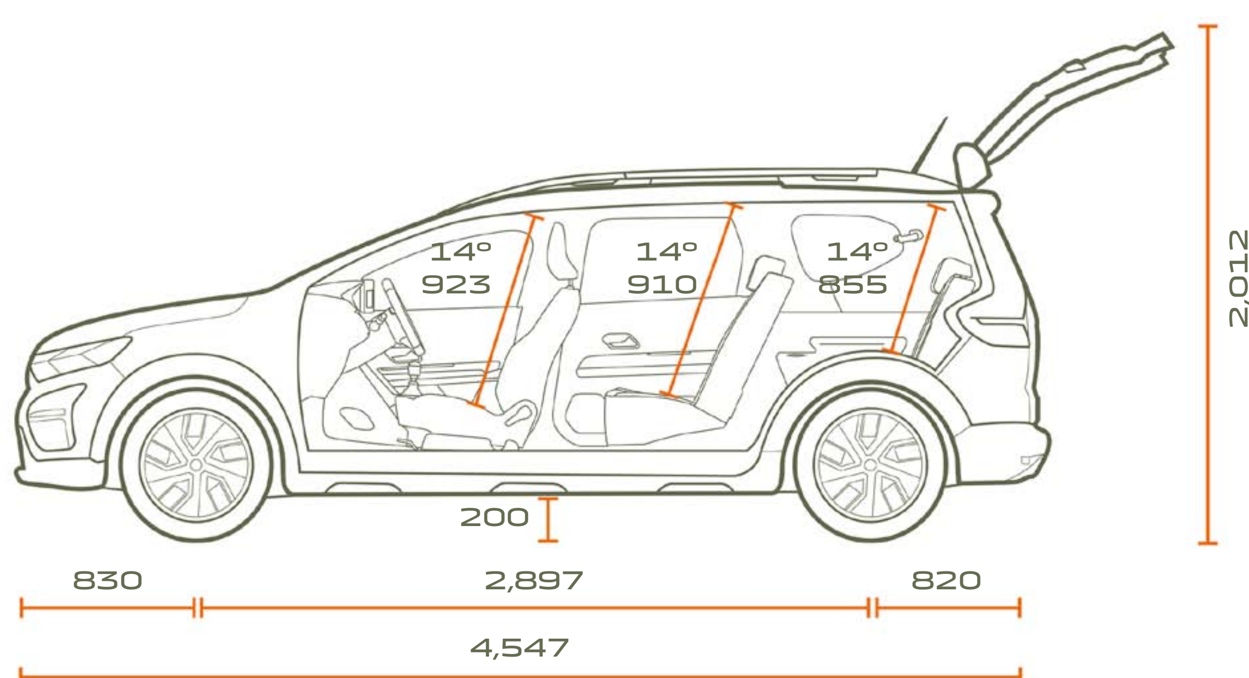
VISTA DE PERFIL 7 LUGARES
