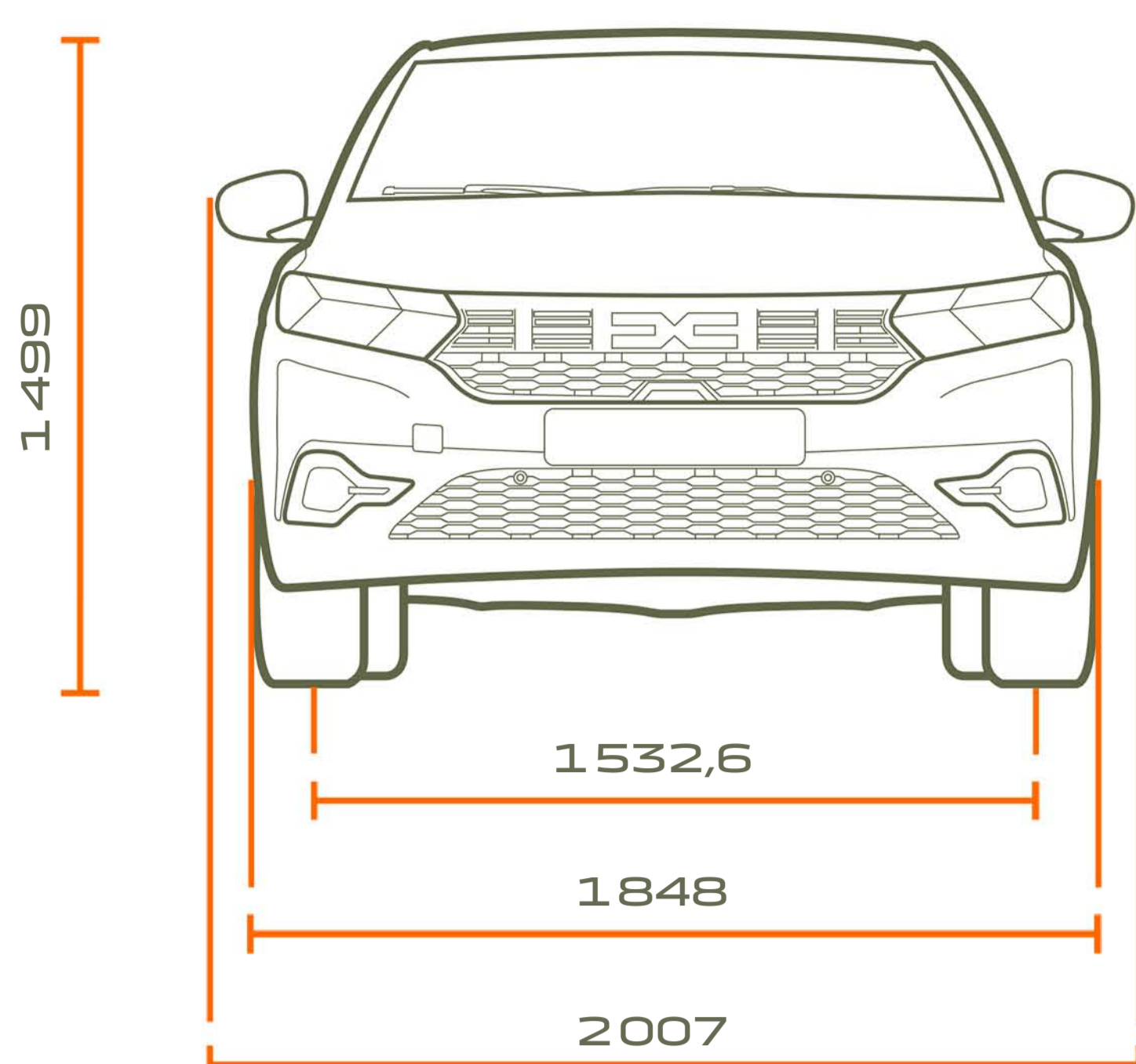
VISTA DIANTEIRA
