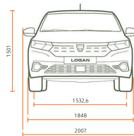
VEDERE FRONTALĂ
