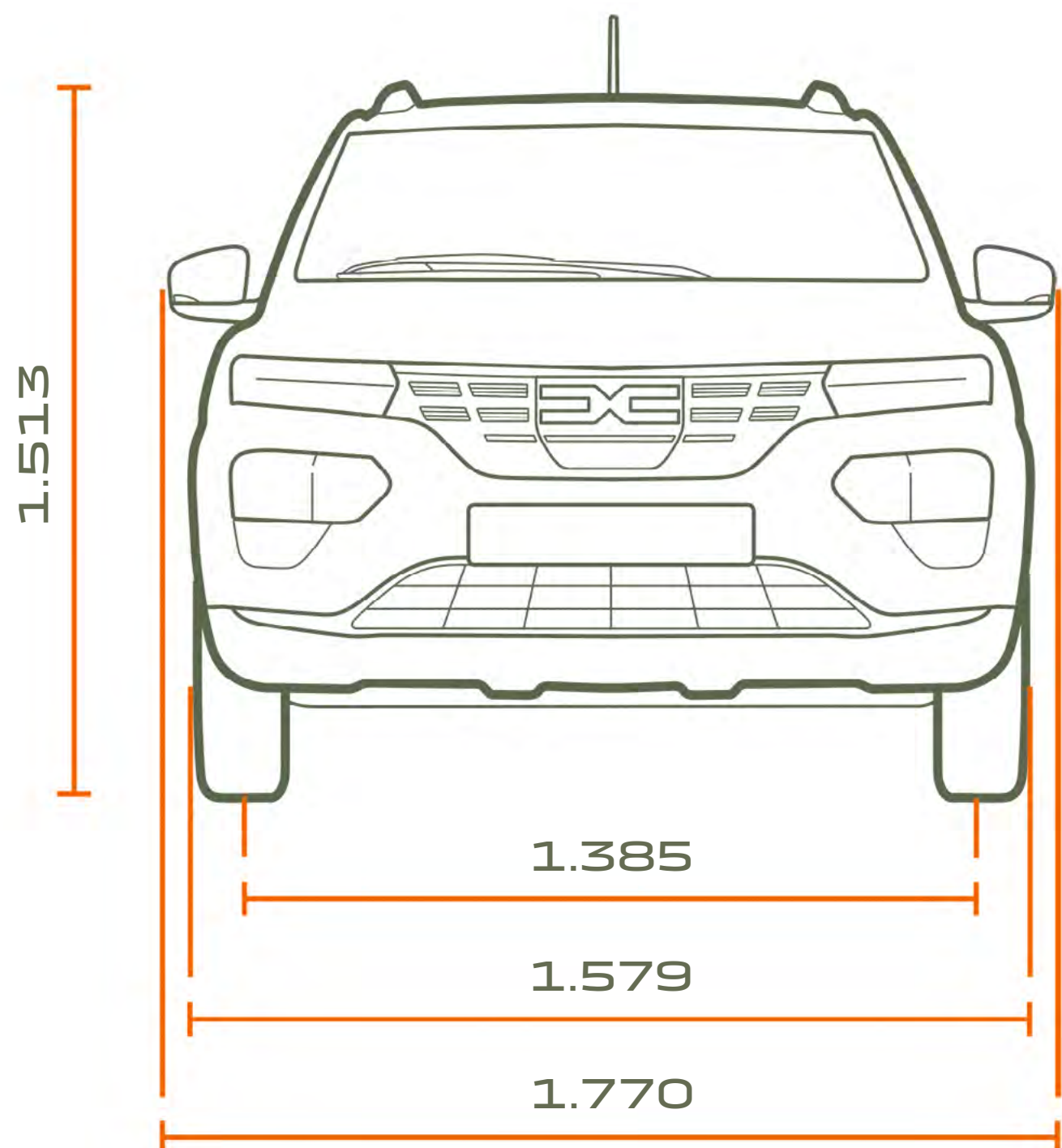
VEDERE FRONTALĂ
