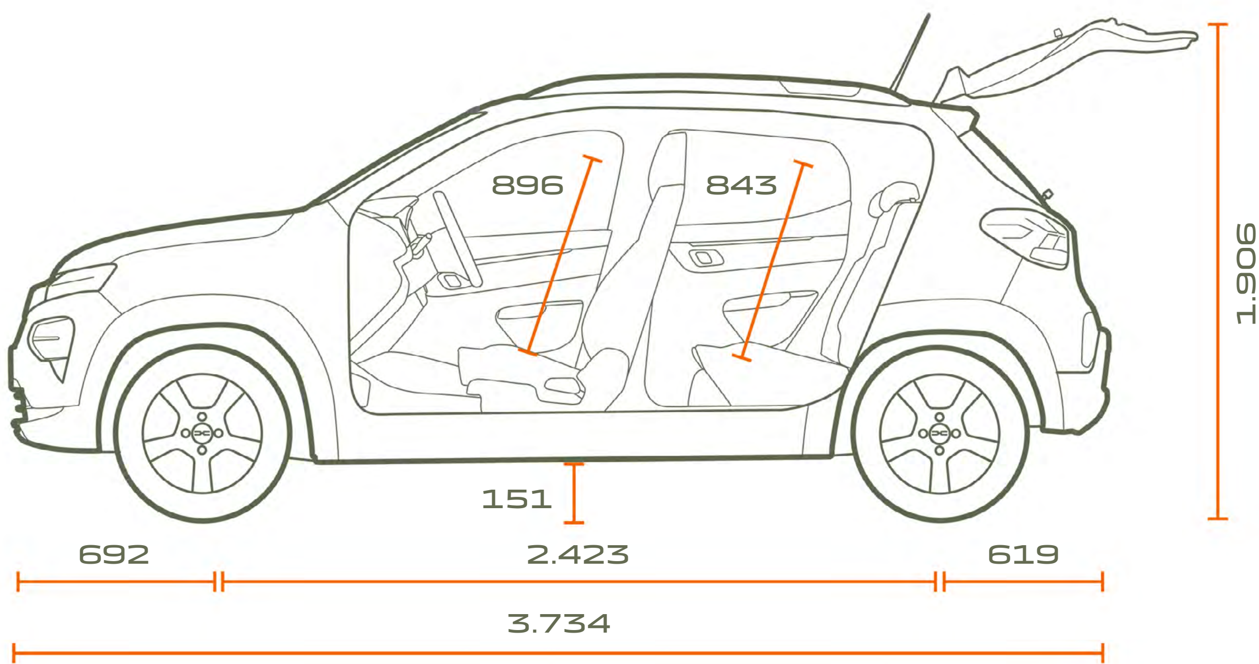
VEDERE LATERALĂ
