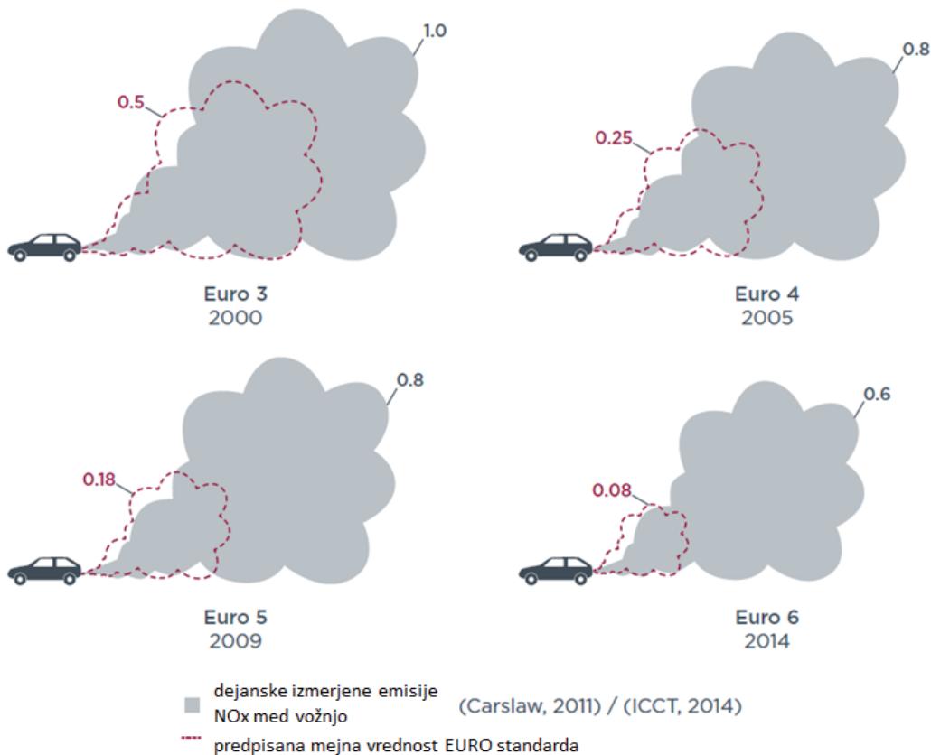
Slika 3 : Dizelska vozila pri vožnji v realnih razmerah ne dosegajo predpisanih mejnih vrednosti za nekatera onesnaževala zraka. Mejne vrednosti za dušikove okside (NOx) iz dizelskih vozil so se od leta 2000 (EURO 3) do leta 2014 (EURO 6) zmanjšale za 85 %. Dejanske emisije NOx v realnih pogojih vožnje pa so se v tem obdobju zmanjšale le za 40 %. Vir: ICCT.
