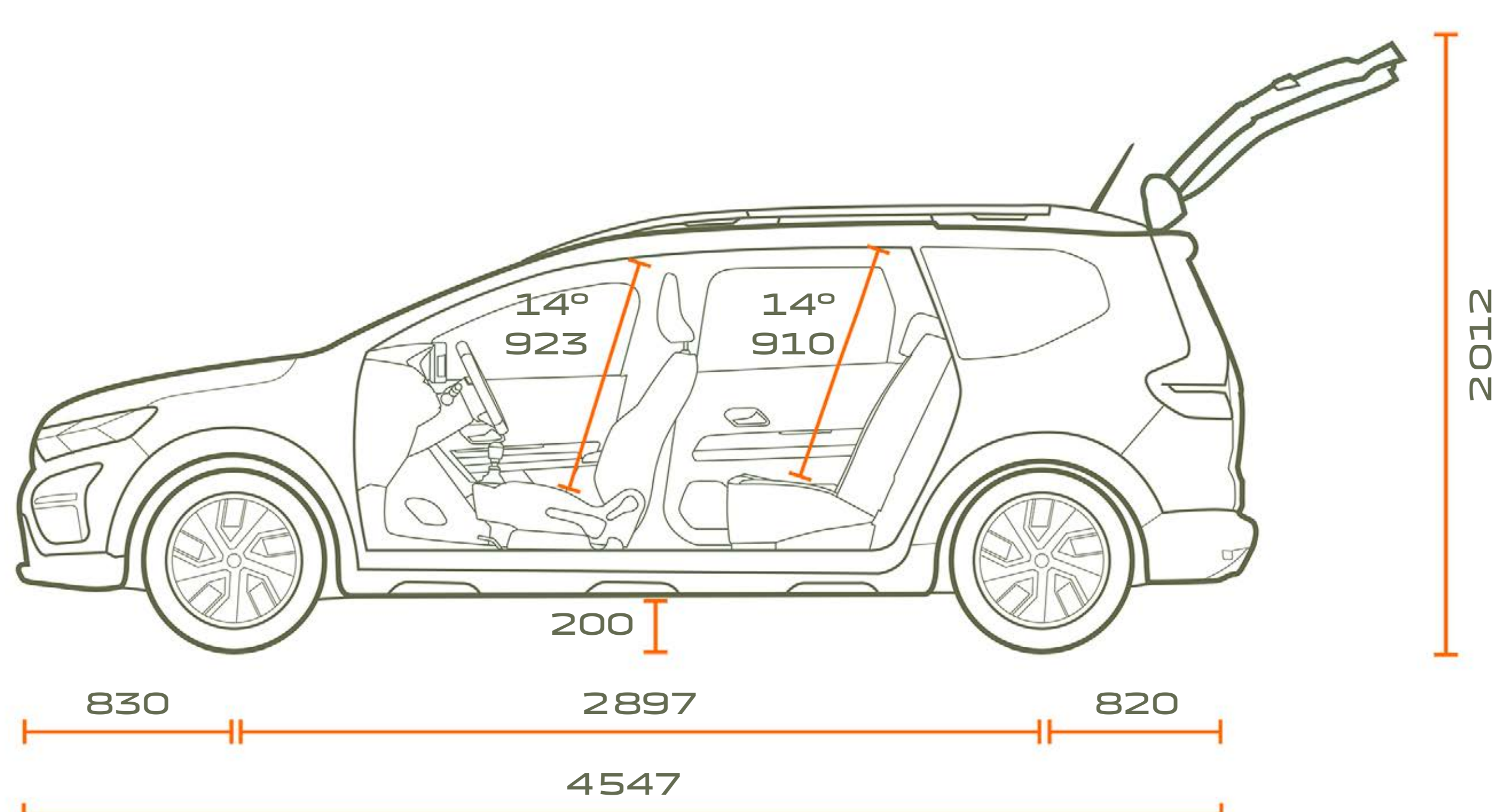
5MIESTNY - BOČNÝ POHĽAD
