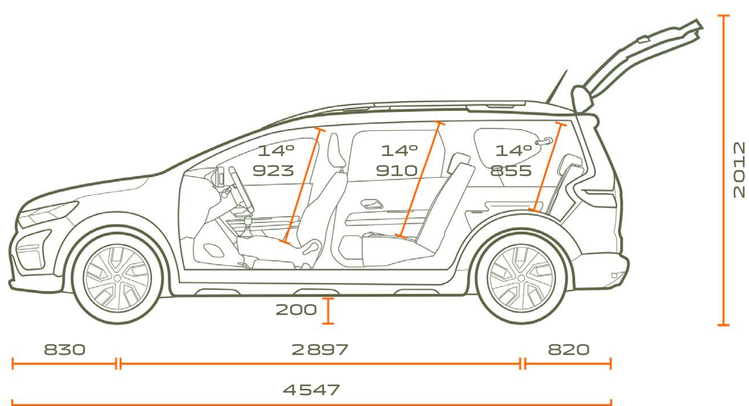
7MIESTNY - BOČNÝ POHĽAD
