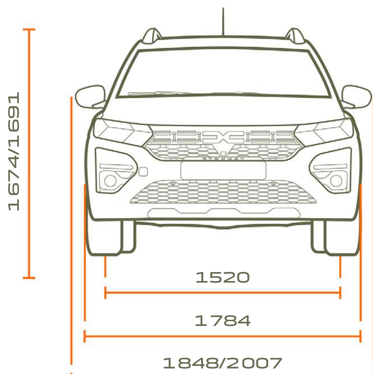
ČELNÝ POHĽAD
