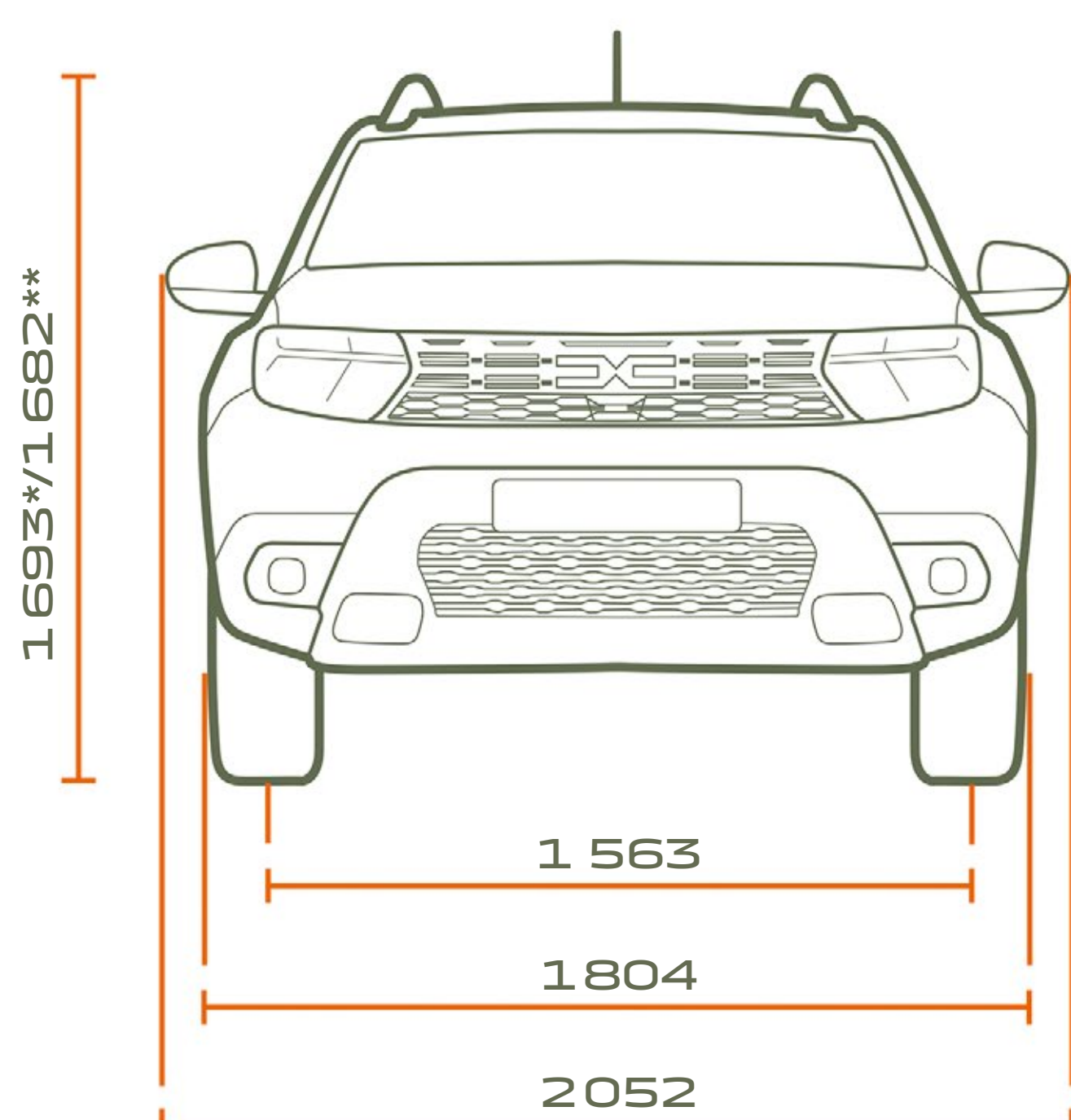
ČELNÝ POHĽAD
