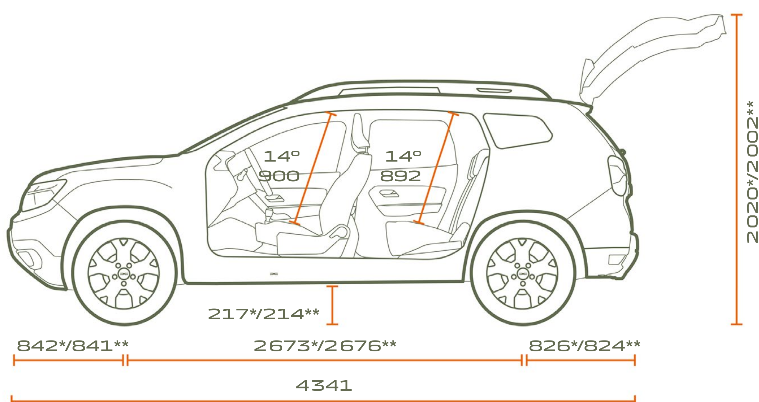
BOČNÝ POHĽAD
