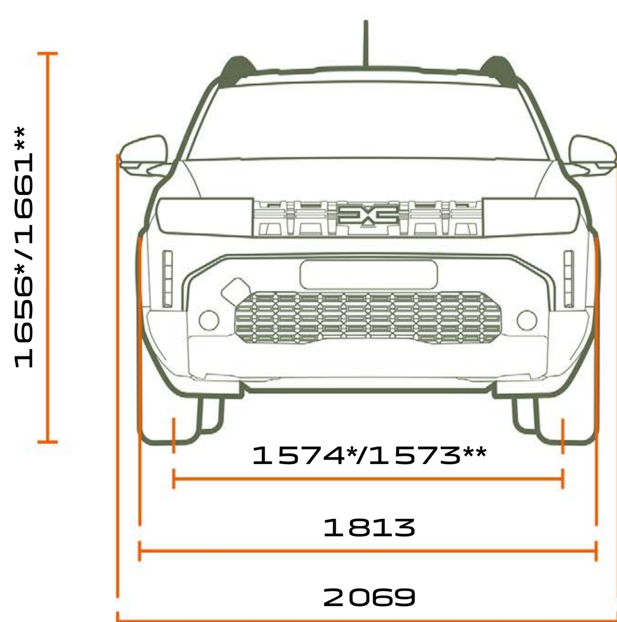
ČELNÝ POHĽAD
