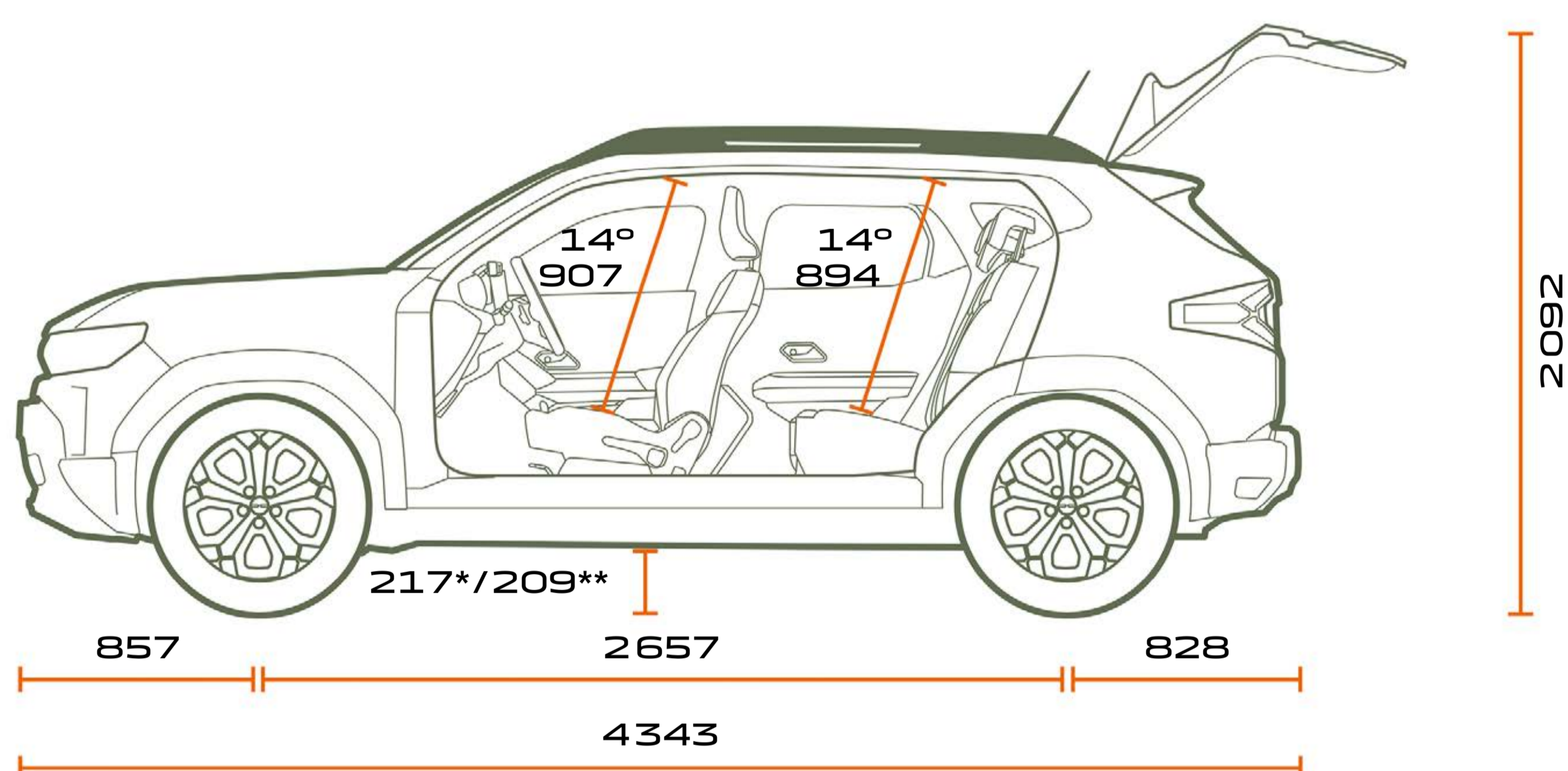
BOČNÝ POHĽAD
