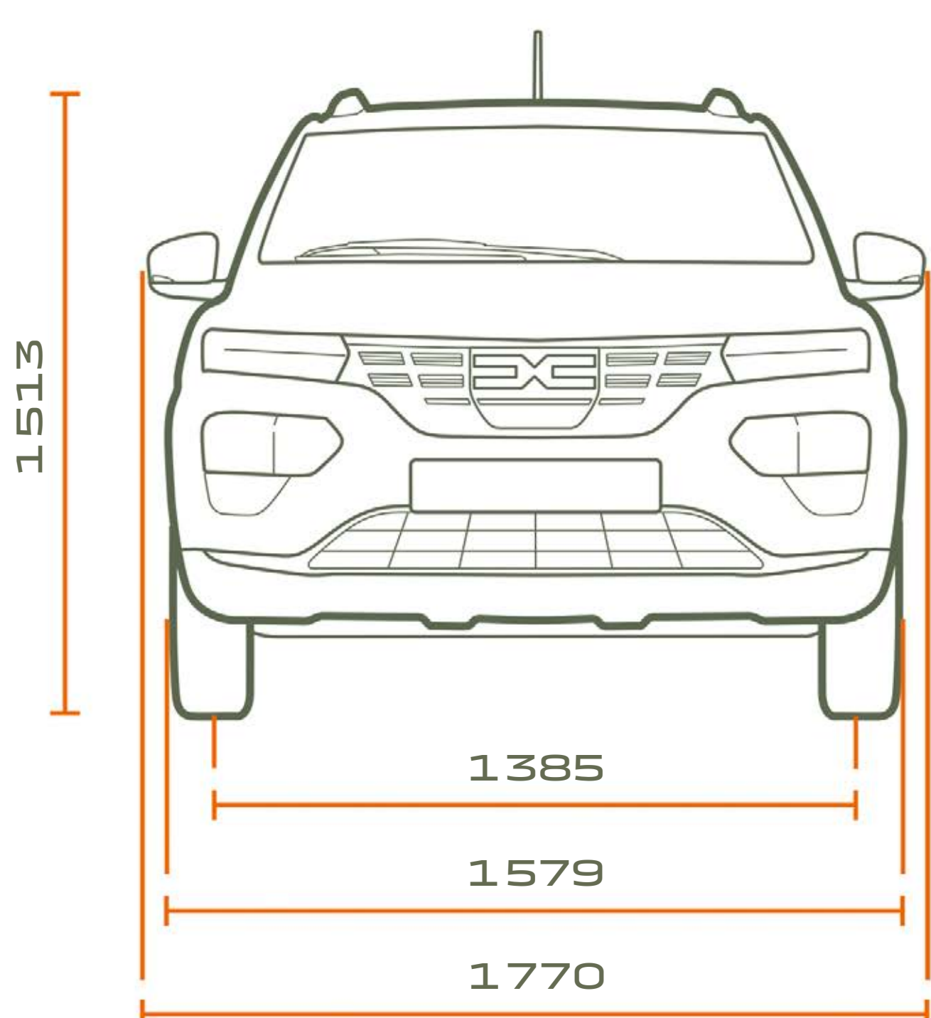
ČELNÝ POHĽAD
