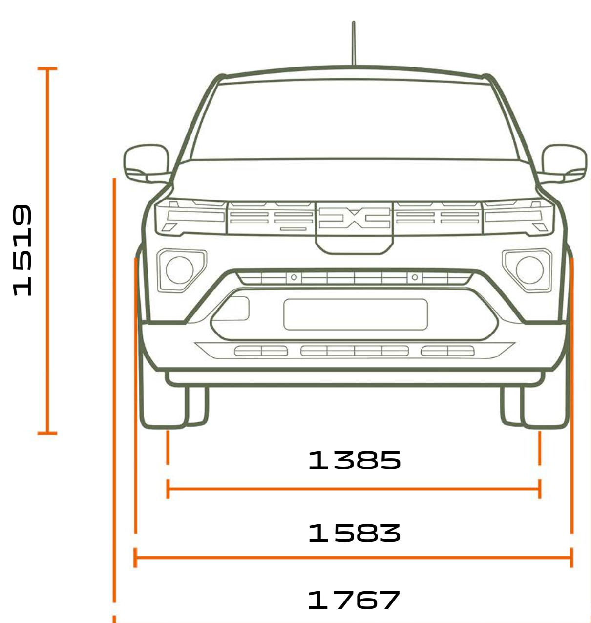
ČELNÝ POHĽAD
