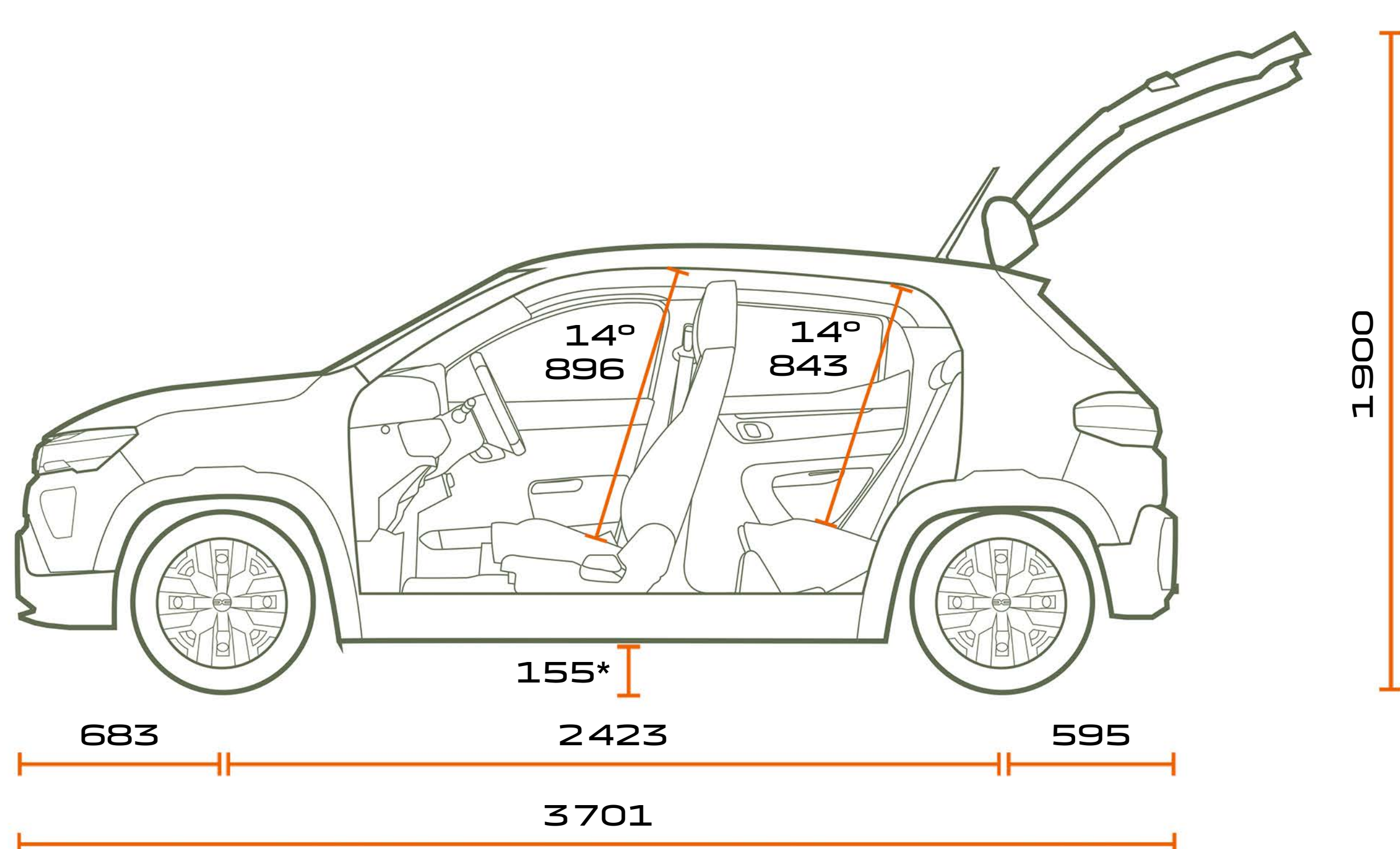
BOČNÝ POHĽAD
