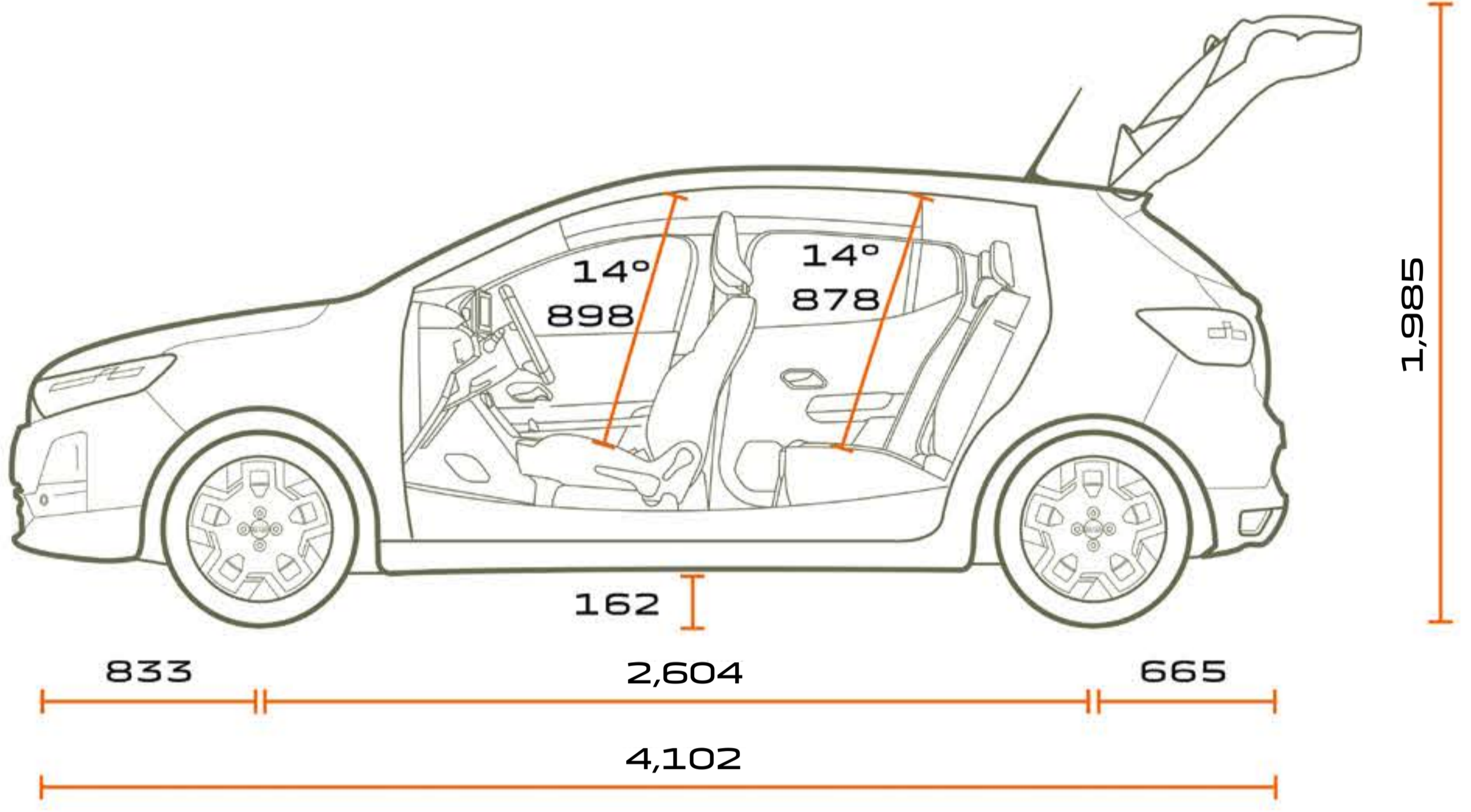
YAN GÖRÜNÜM
