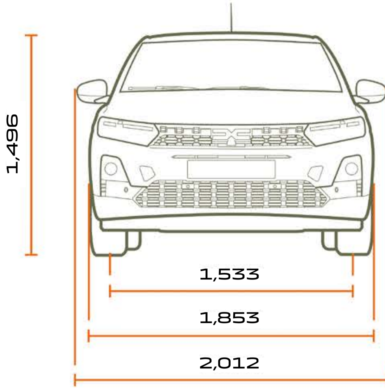
ÖN GÖRÜNÜM
