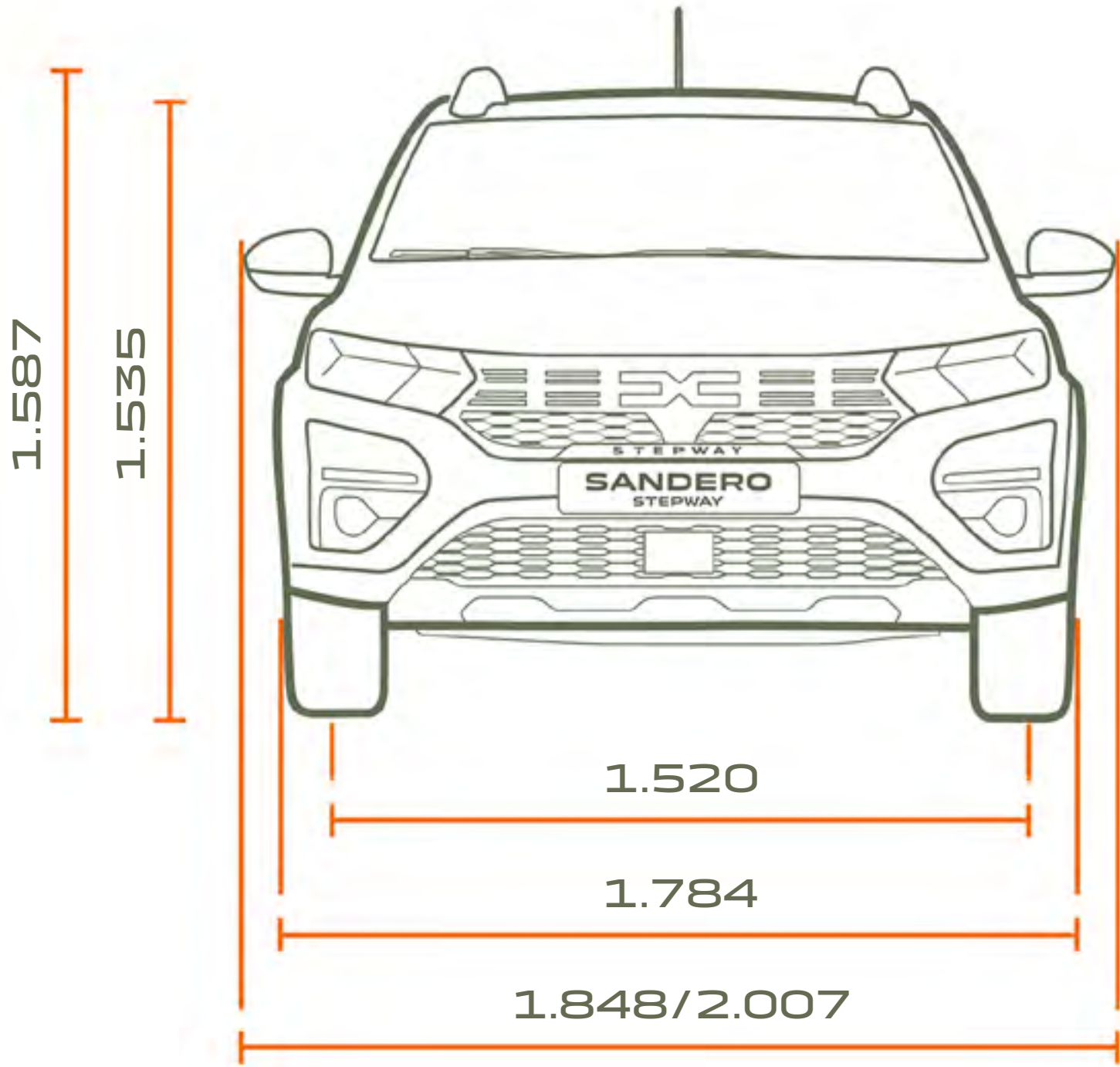
ÖNDEN GÖRÜNÜM
