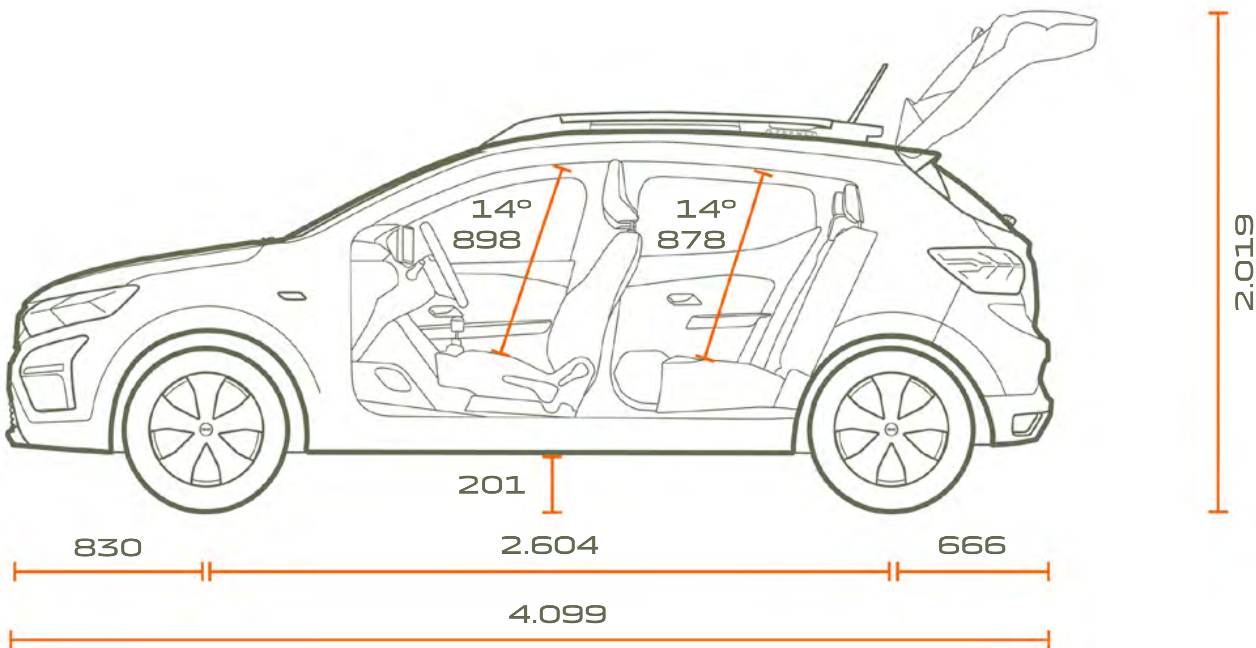
YANDAN GÖRÜNÜM
