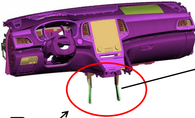
Verstärkungen beidseitig unter der Mittelkonsole
