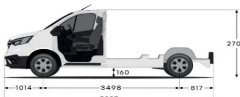
Chassi-platta
